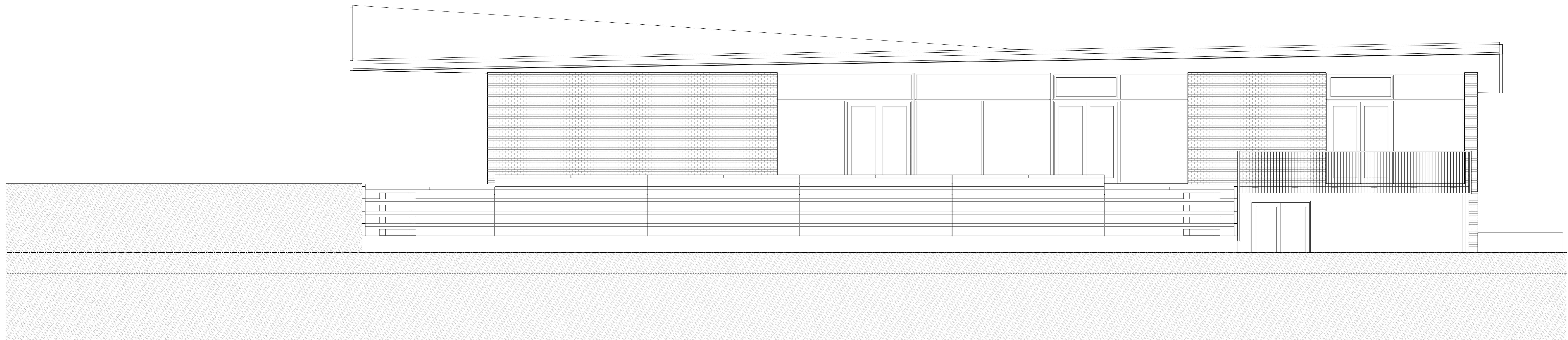
GEVELAANZICHT ZUIDZIJDE
