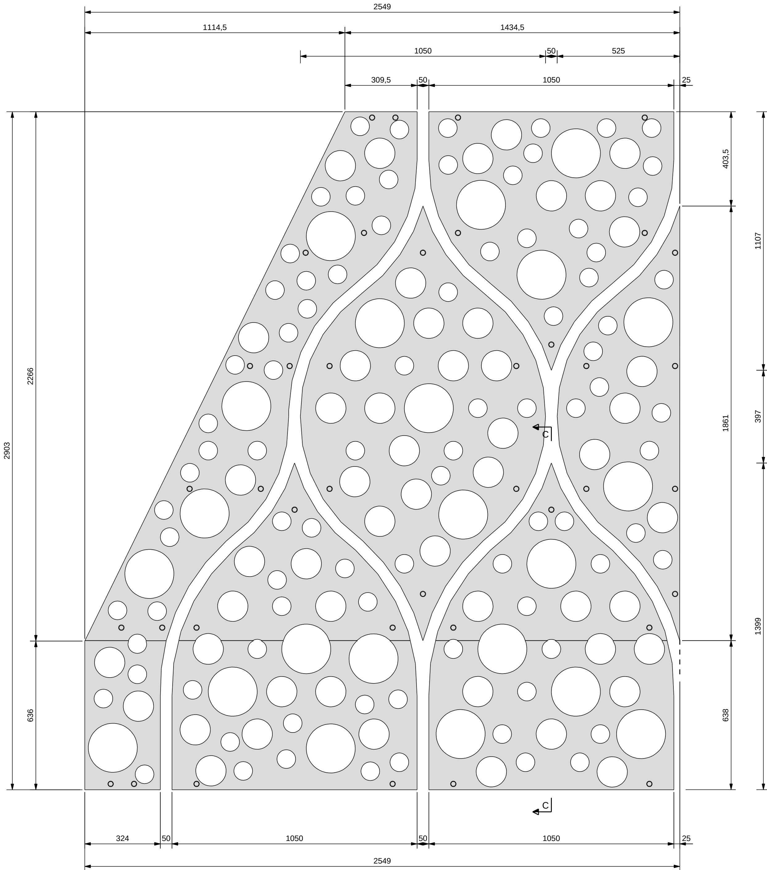
RECHTER AANZICHT (VOORPLAAT) - UITSLAG
