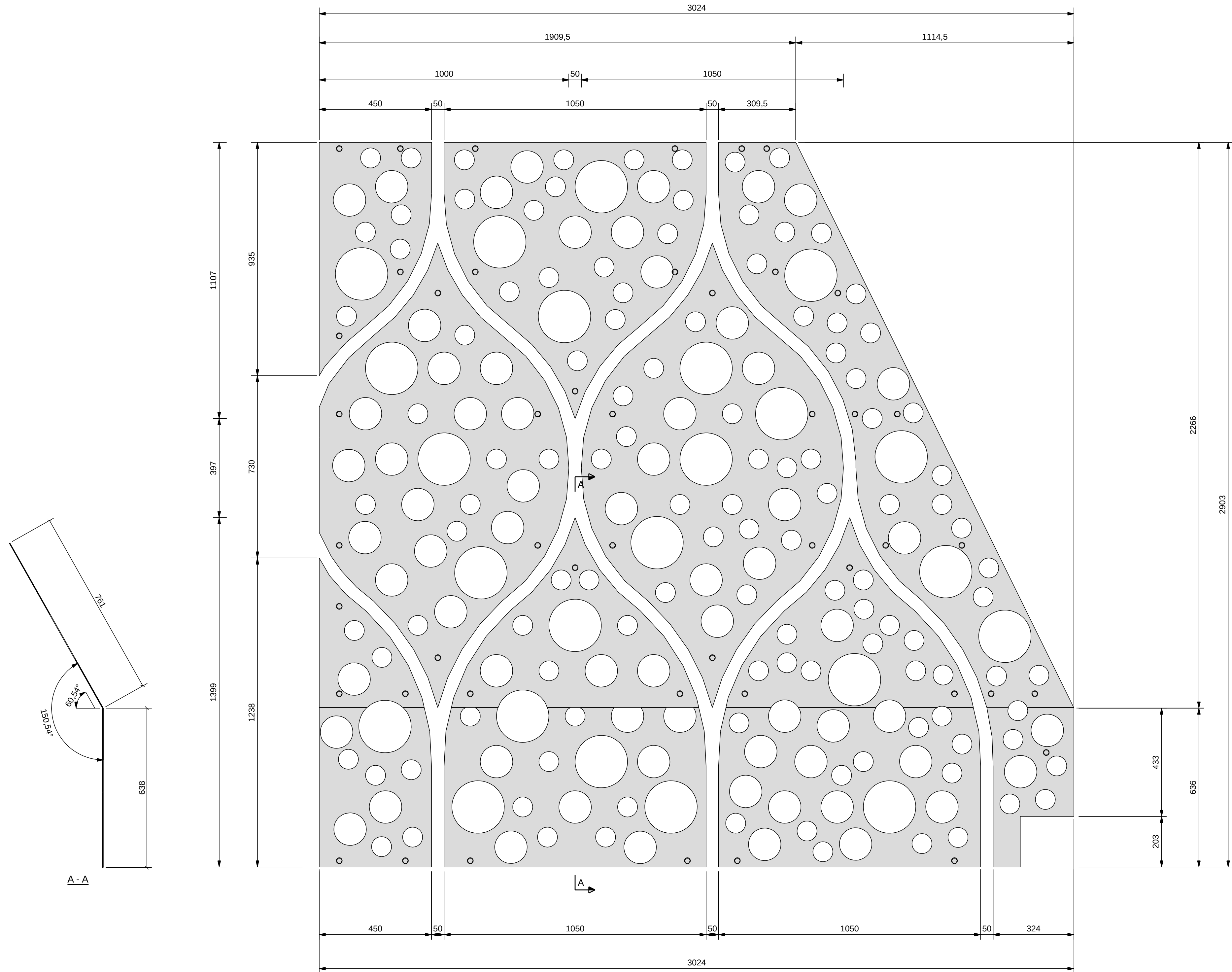
LINKER AANZICHT (VOORPLAAT) - UITSLAG
