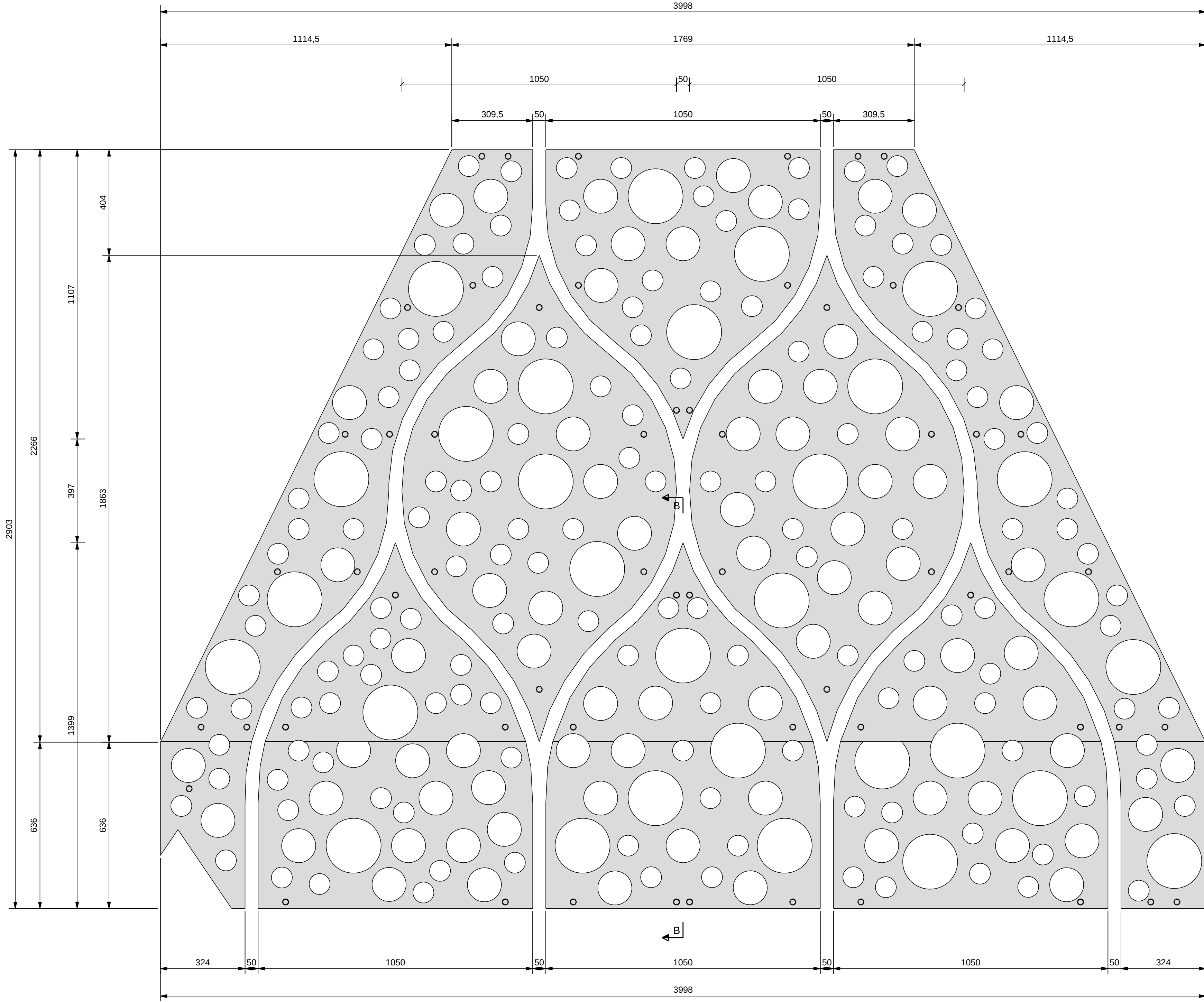
VOOR AANZICHT (VOORPLAAT) - UITSLAG
