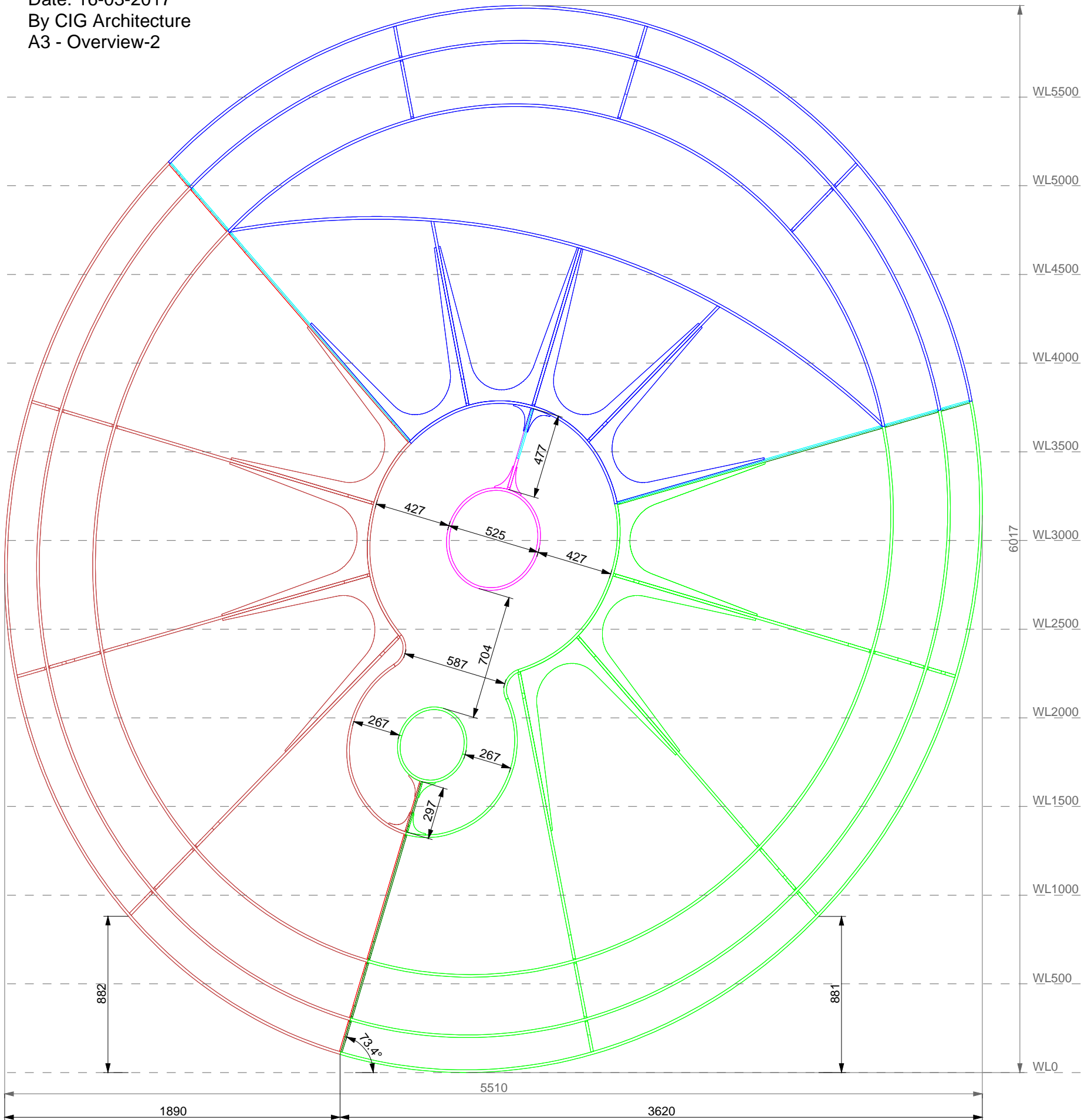
Vooranzicht 1:25
