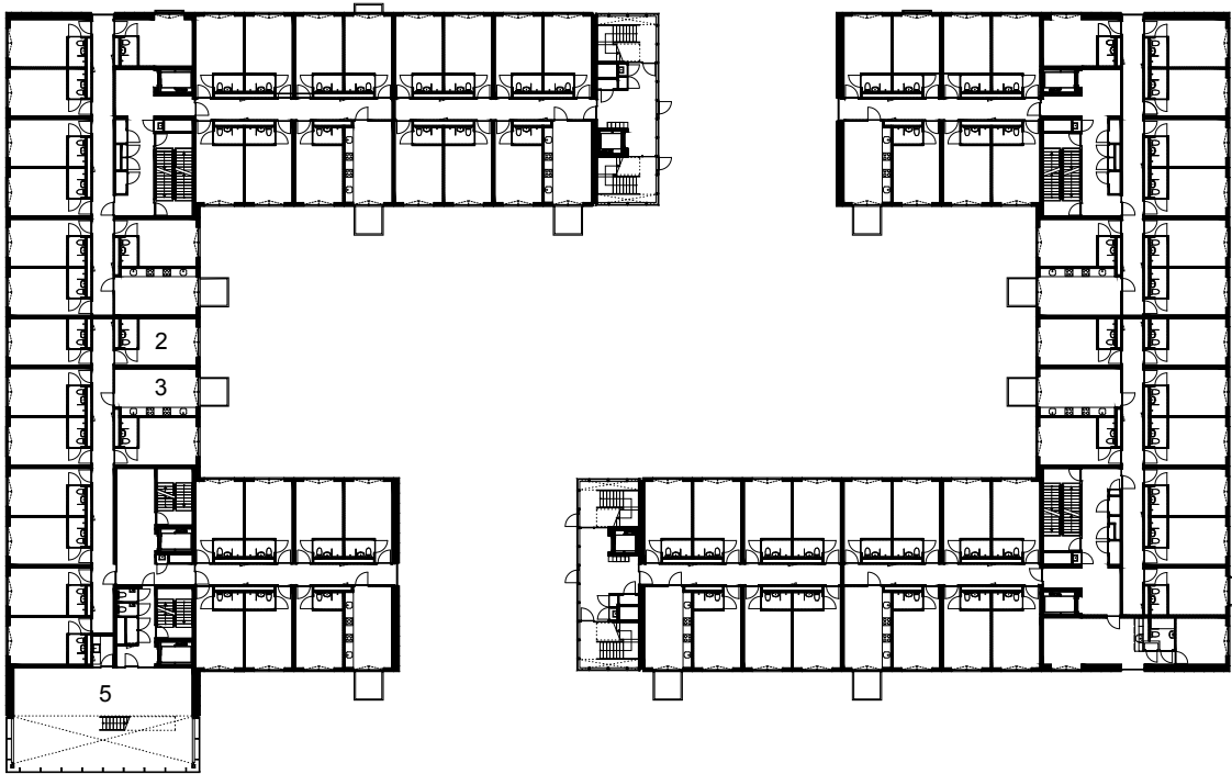
tweede verdieping
