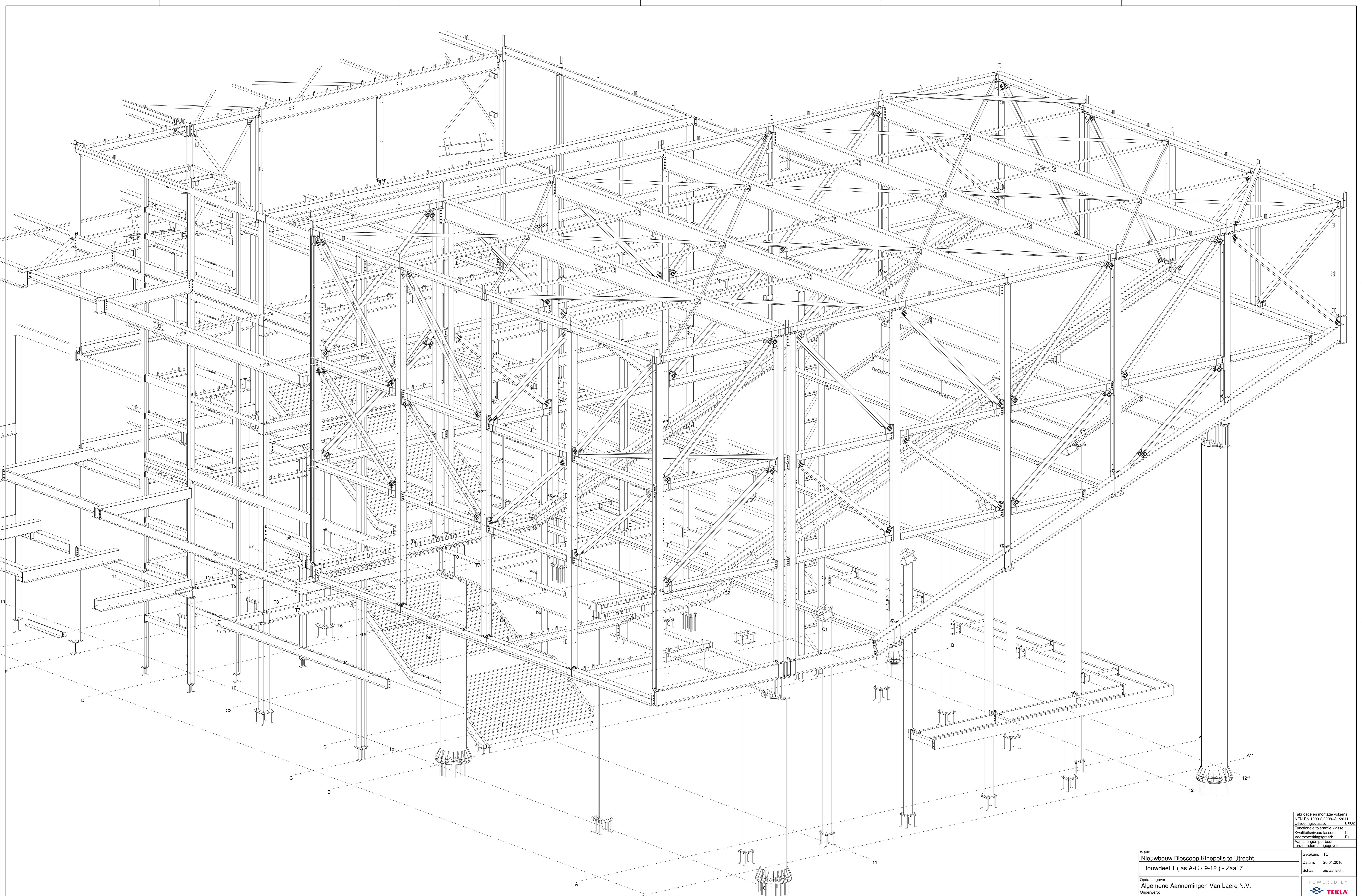
A-ØD-Merkenoverzicht 1:45
