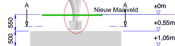
Aanzicht kijkend naar TU-gebouw Fundering ligt in lijn met de lijnen van de gebouwen
