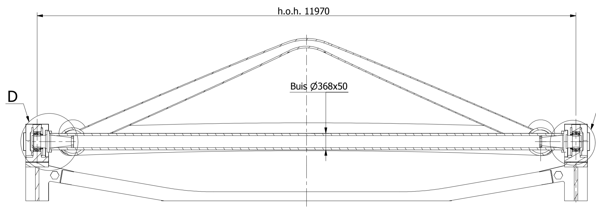
Doorsnede A-A Draaipunt Balans (Schaal 1 : 50)
