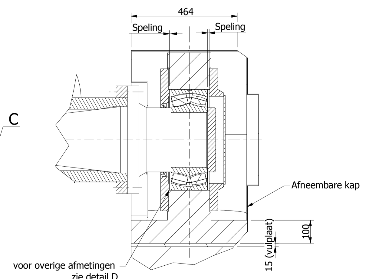
Detail C Los lager (Schaal 1 : 10)
