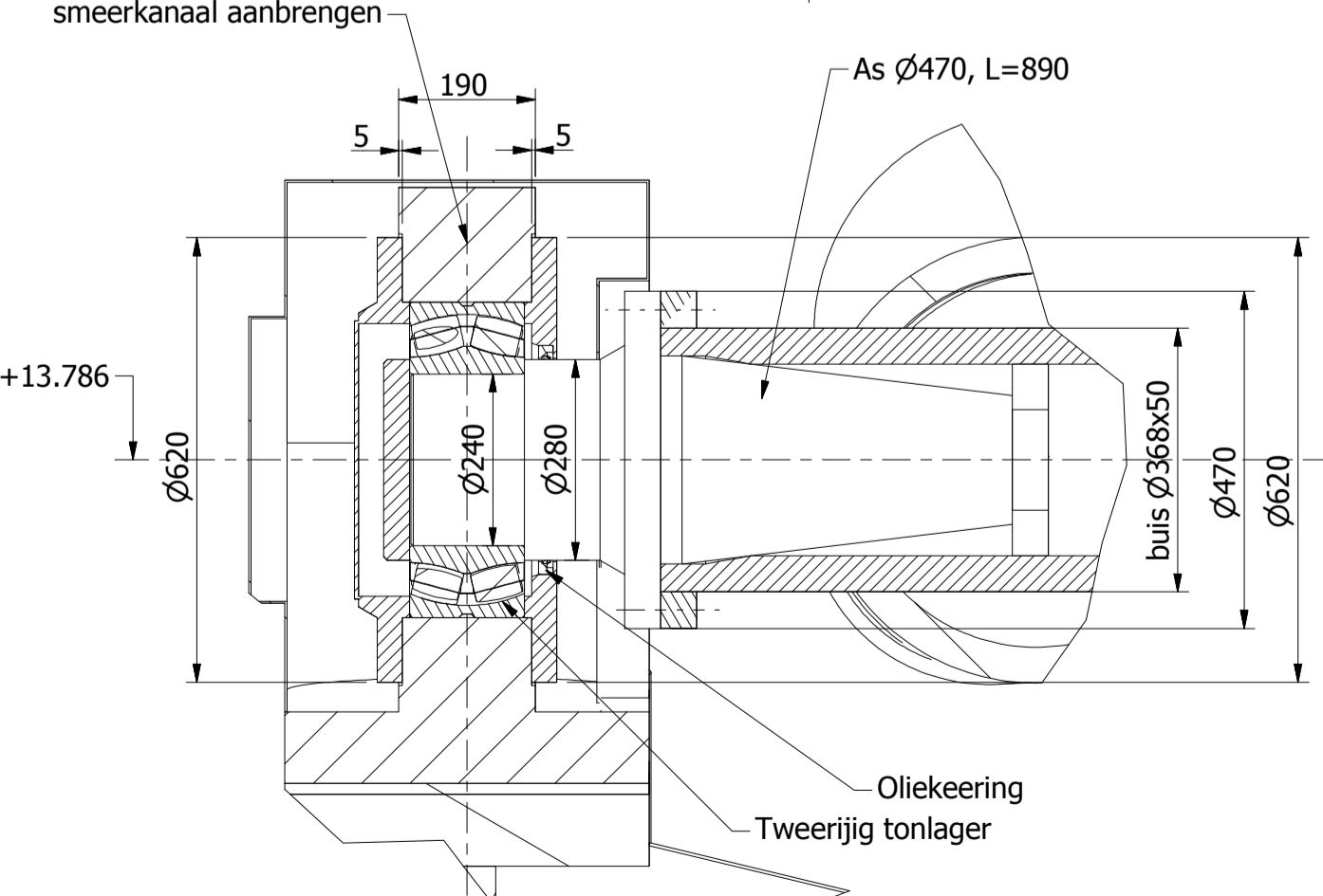
Detail D Vast lager (Schaal 1 : 10)
