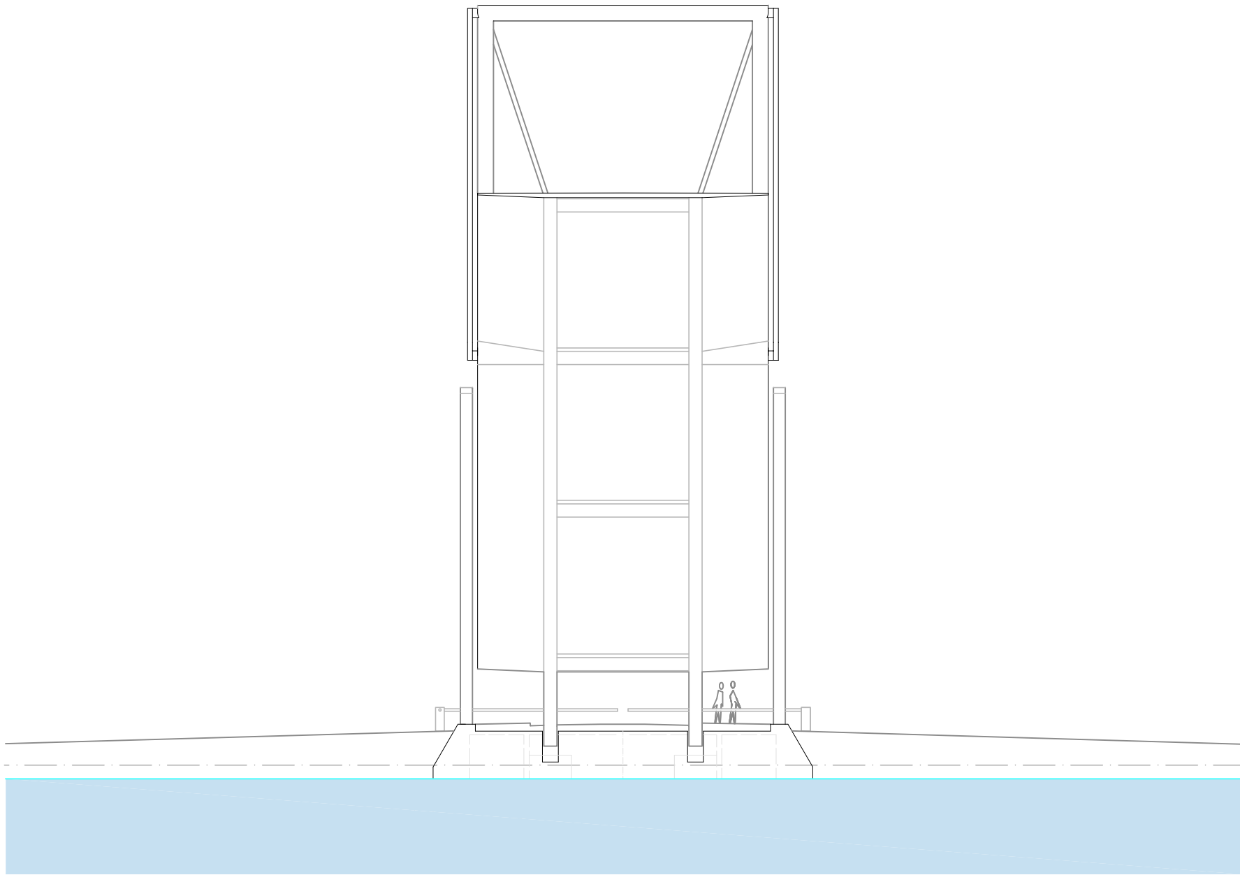
aanzicht vanuit noorden - brug geopend
