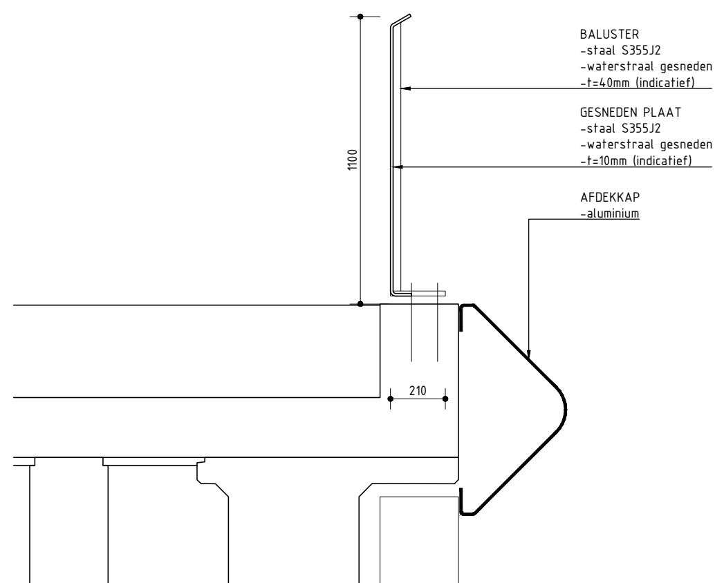
VARIANT 3 SCHAAL 1:20
