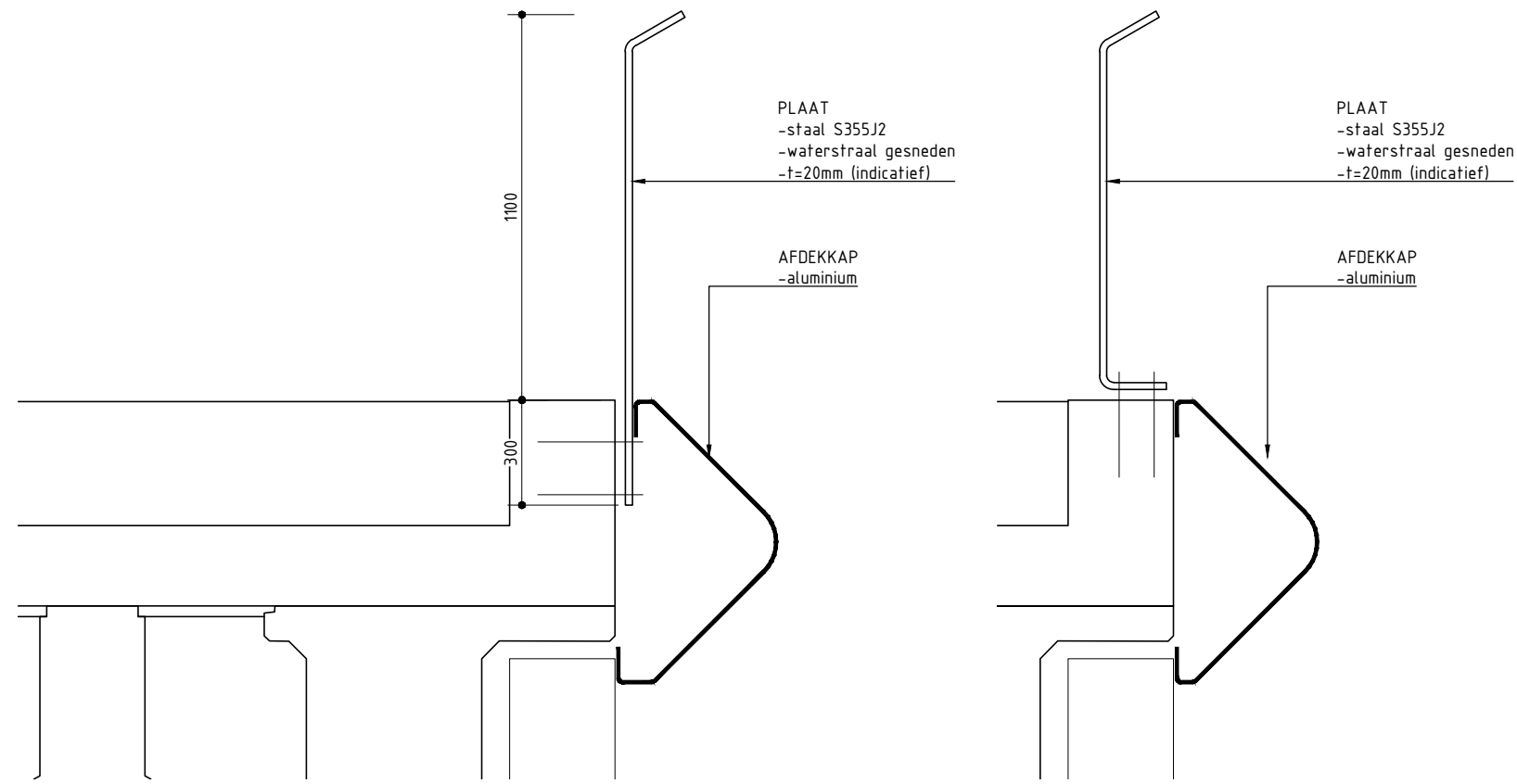
VARIANT 1 SCHAAL 1:20
