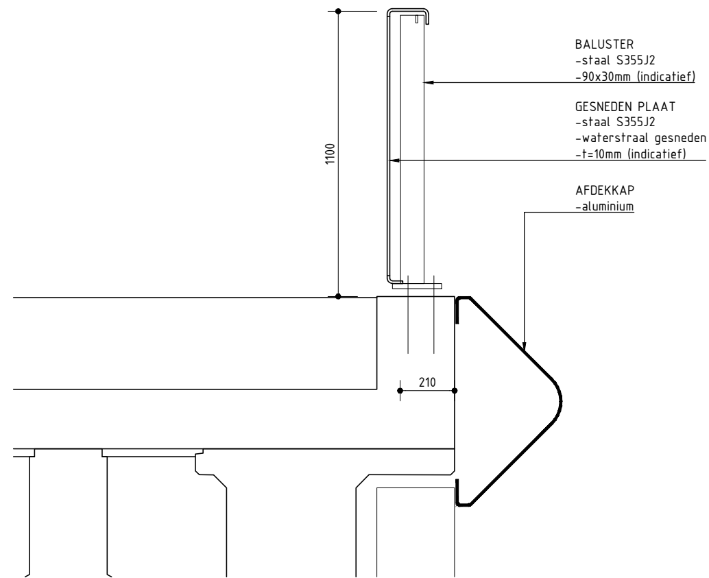
VARIANT 2 SCHAAL 1:20
