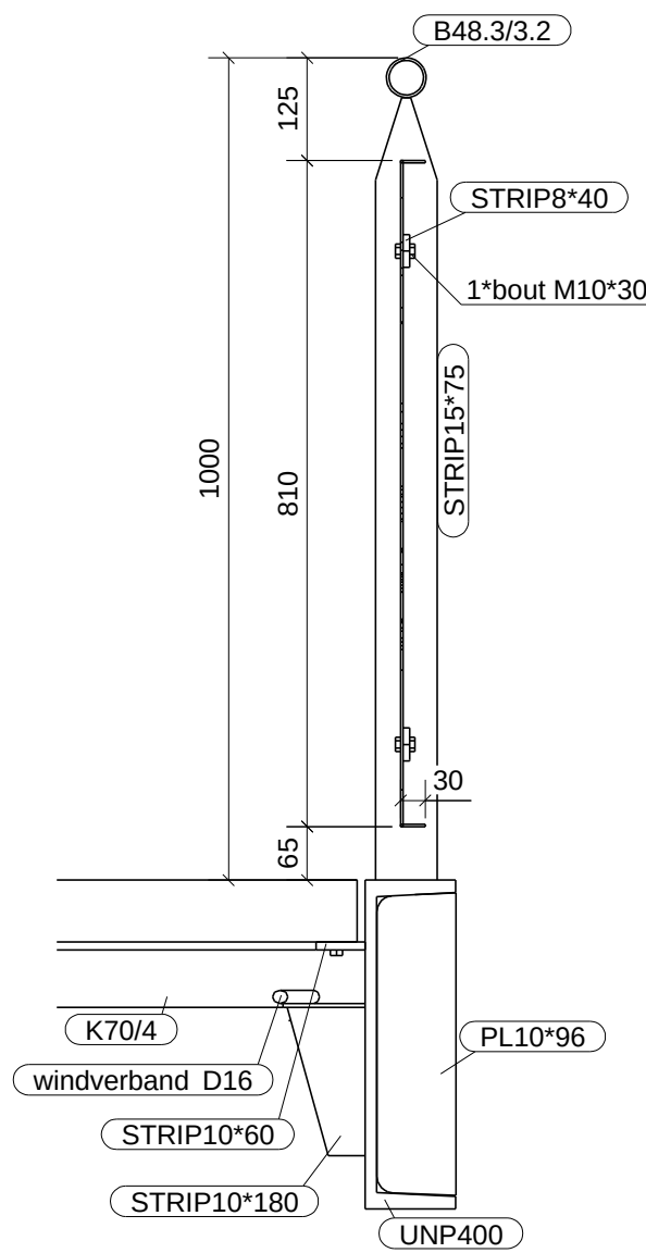
dsn B - B, 1:10
