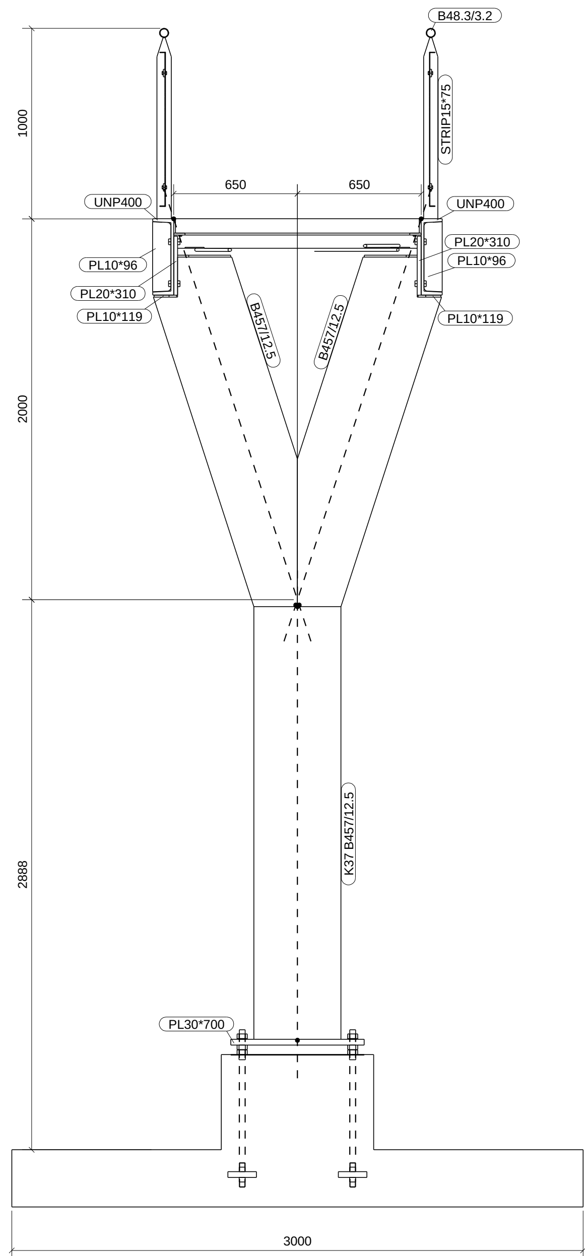
dsn A - A, 1:20
