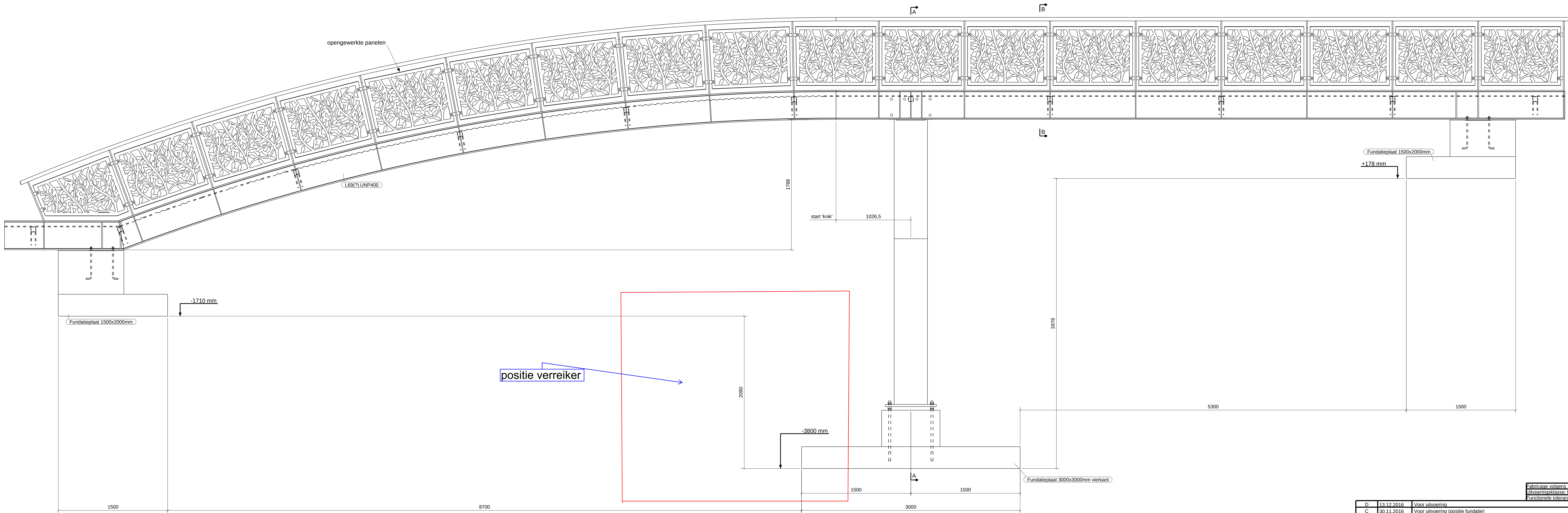
Aanzicht brug
