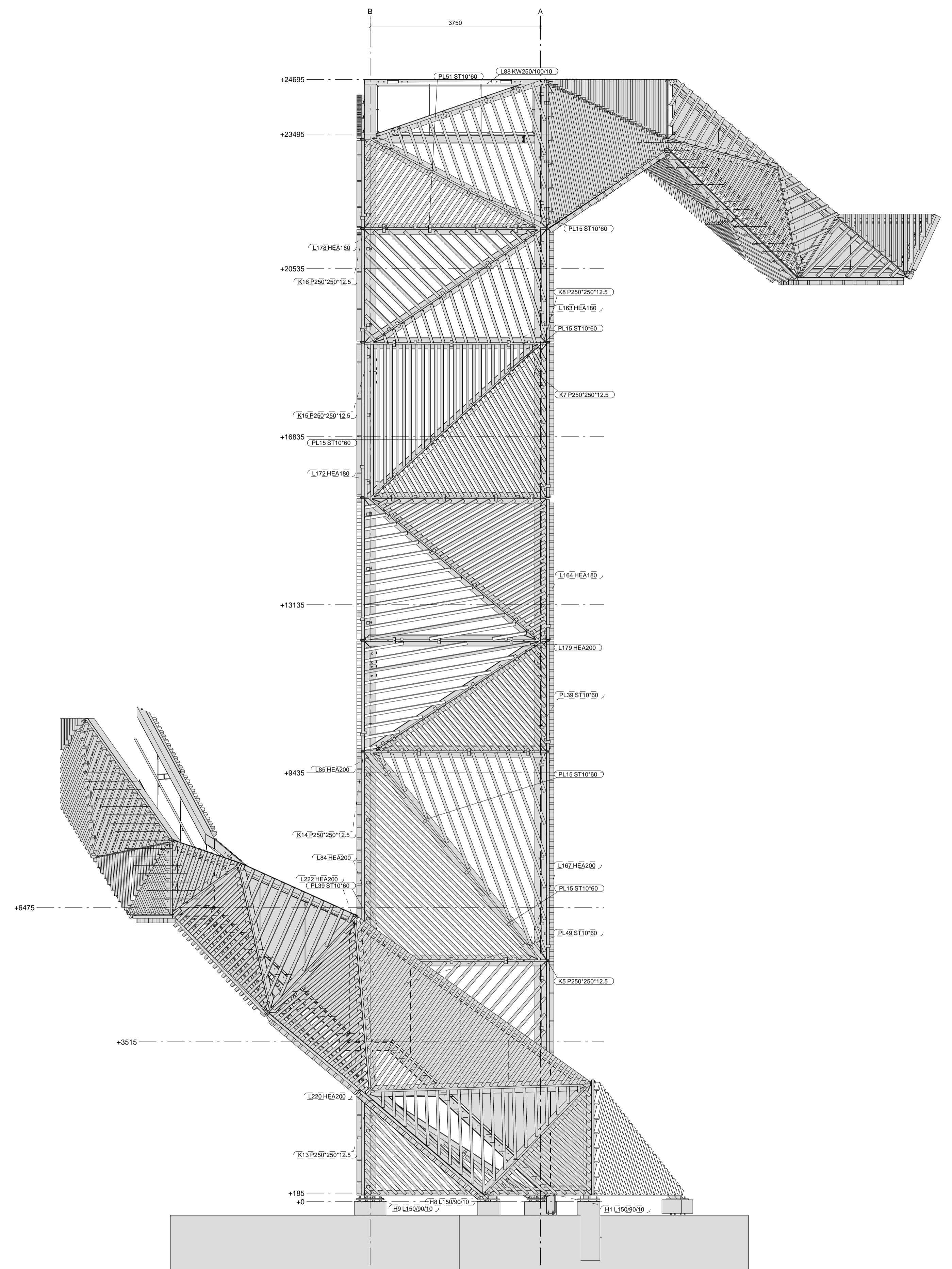
AANZICHT AS 2 1:40
