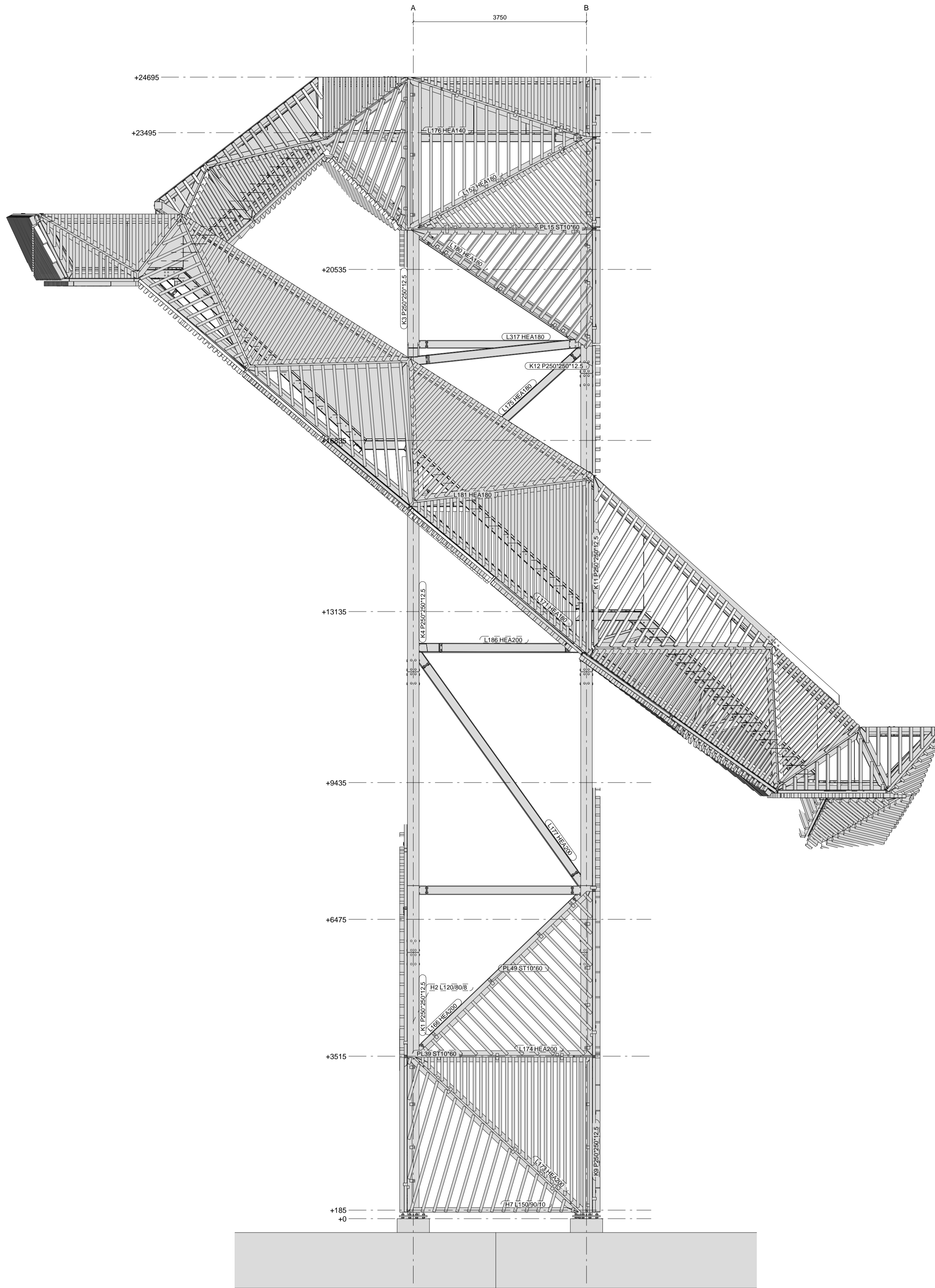
AANZICHT AS 1 1:40
