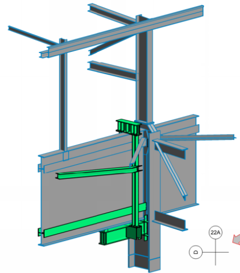
Fase-03 NSSG1_3D console plaatligger dak
