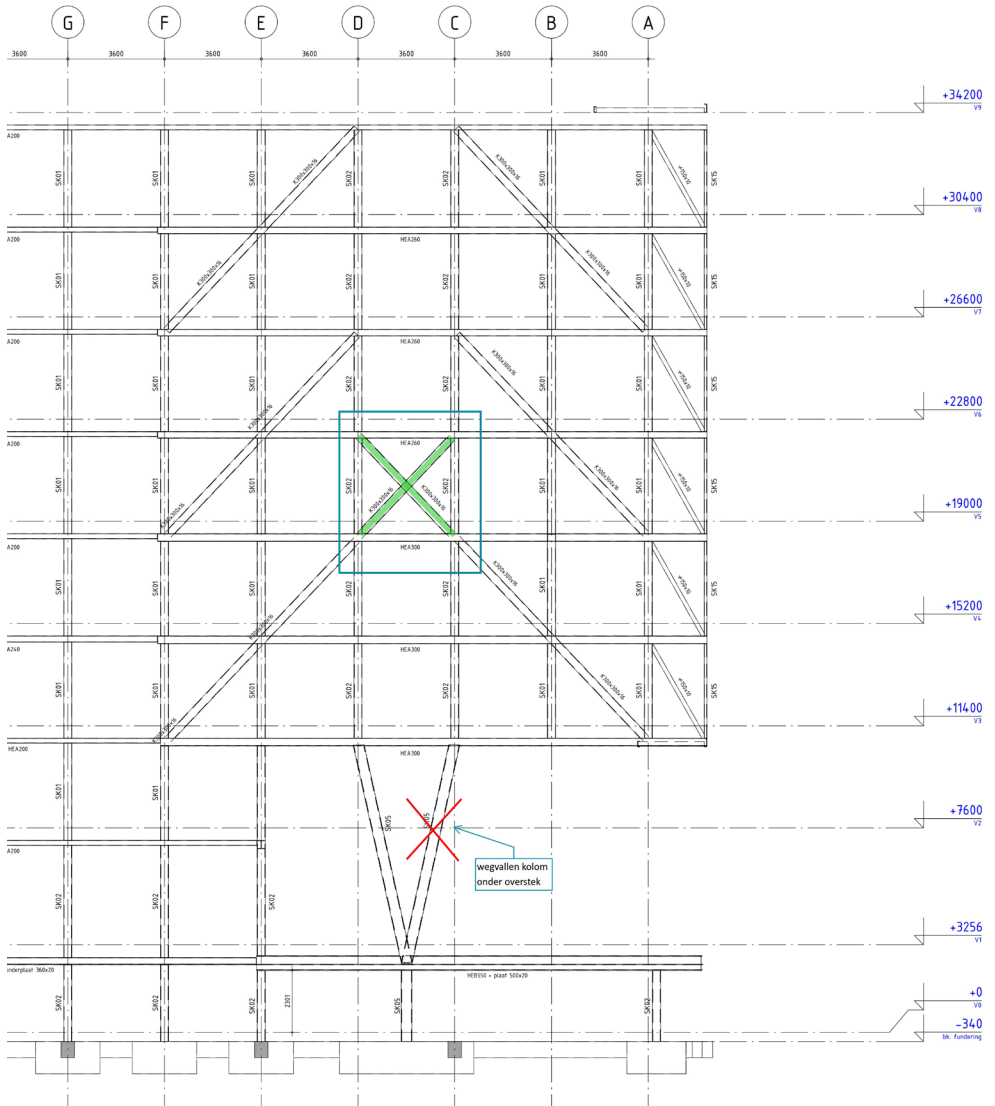
STC Waalhaven z.z. 16 - 2e draagweg - wegvallen kolommen as 1 en 4 (2) - Pieters Bouwtechniek
