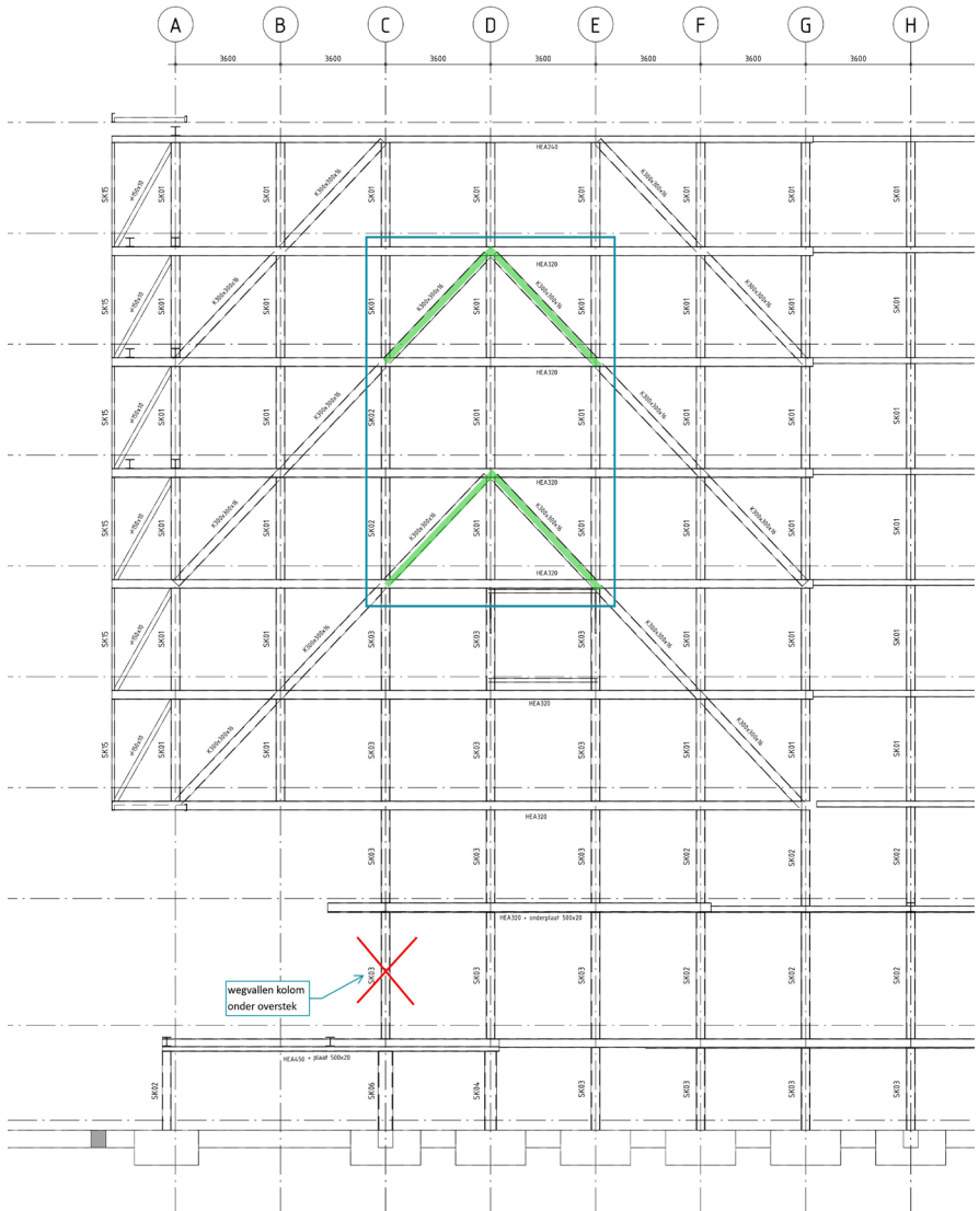
STC Waalhaven z.z. 16 - 2e draagweg - wegvallen kolommen as 1 en 4 (1) - Pieters Bouwtechniek
