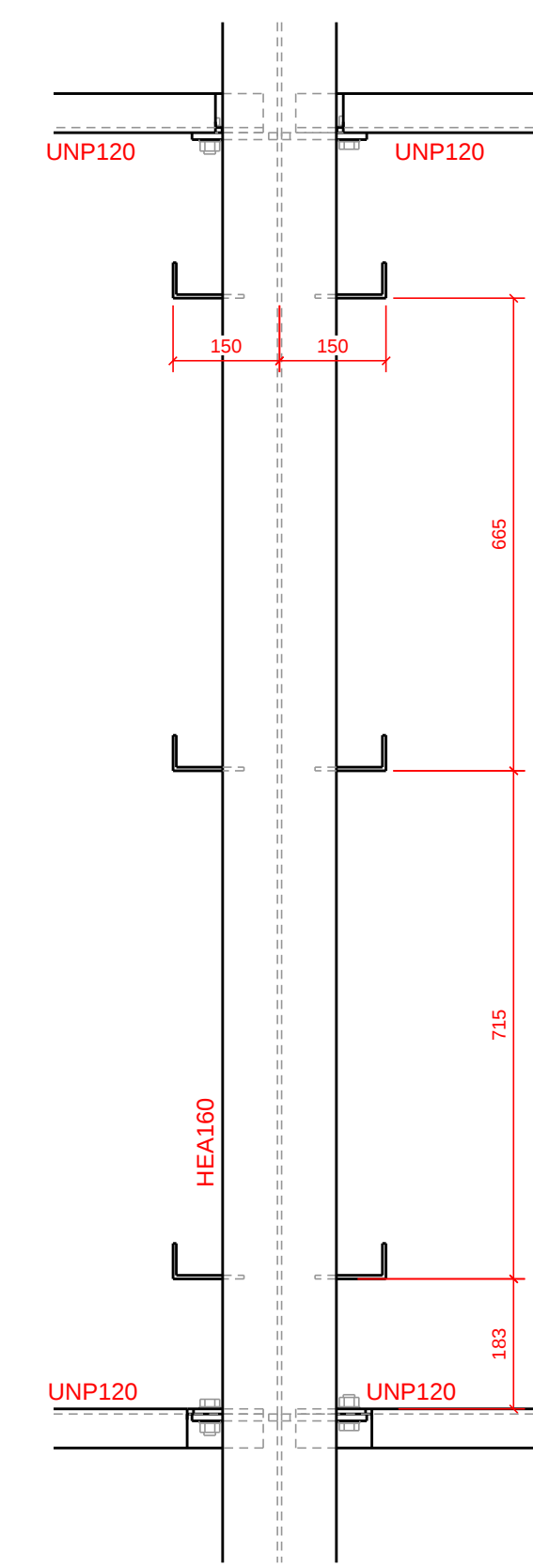
Typical maatvoering 3 bouwkundige hoeklijnen
