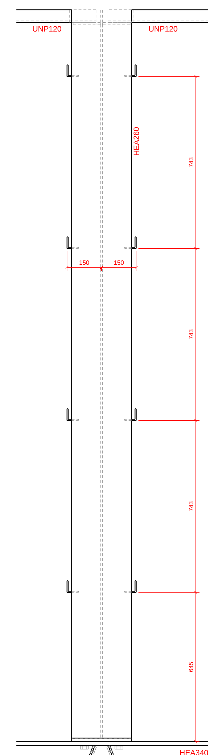
Typical maatvoering 4 bouwkundige hoeklijnen
