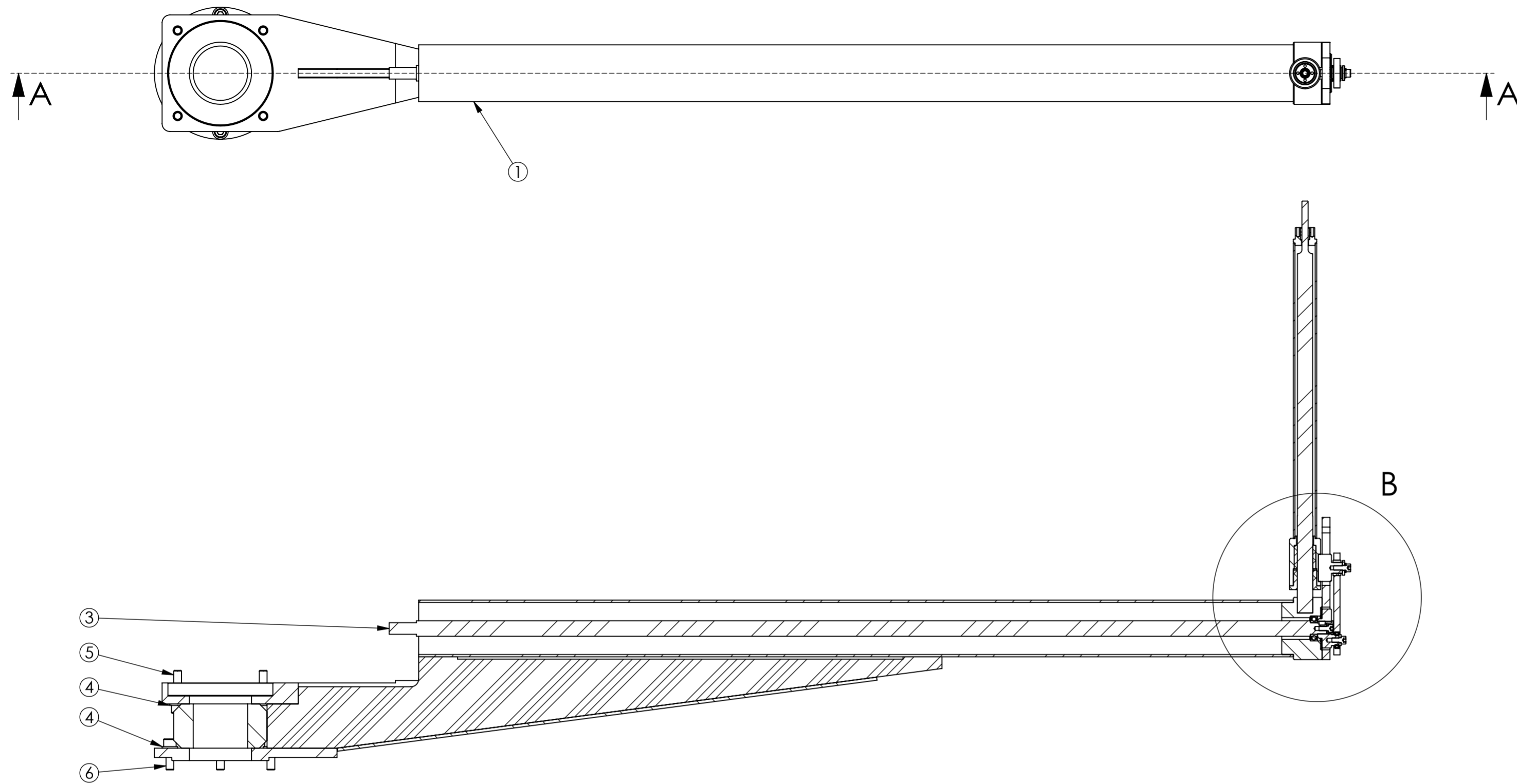
SECTION A-A
