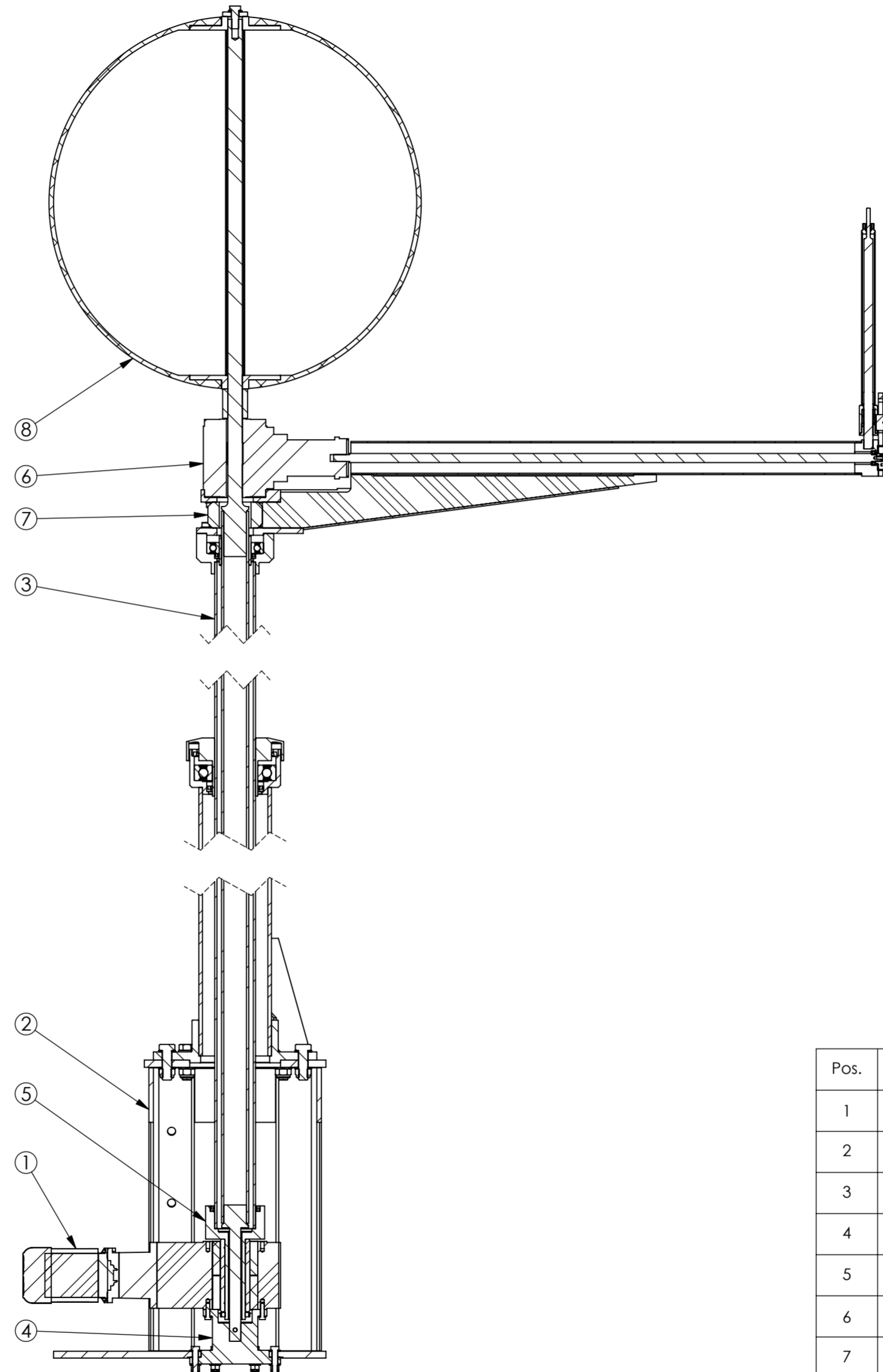
SECTION A-A
