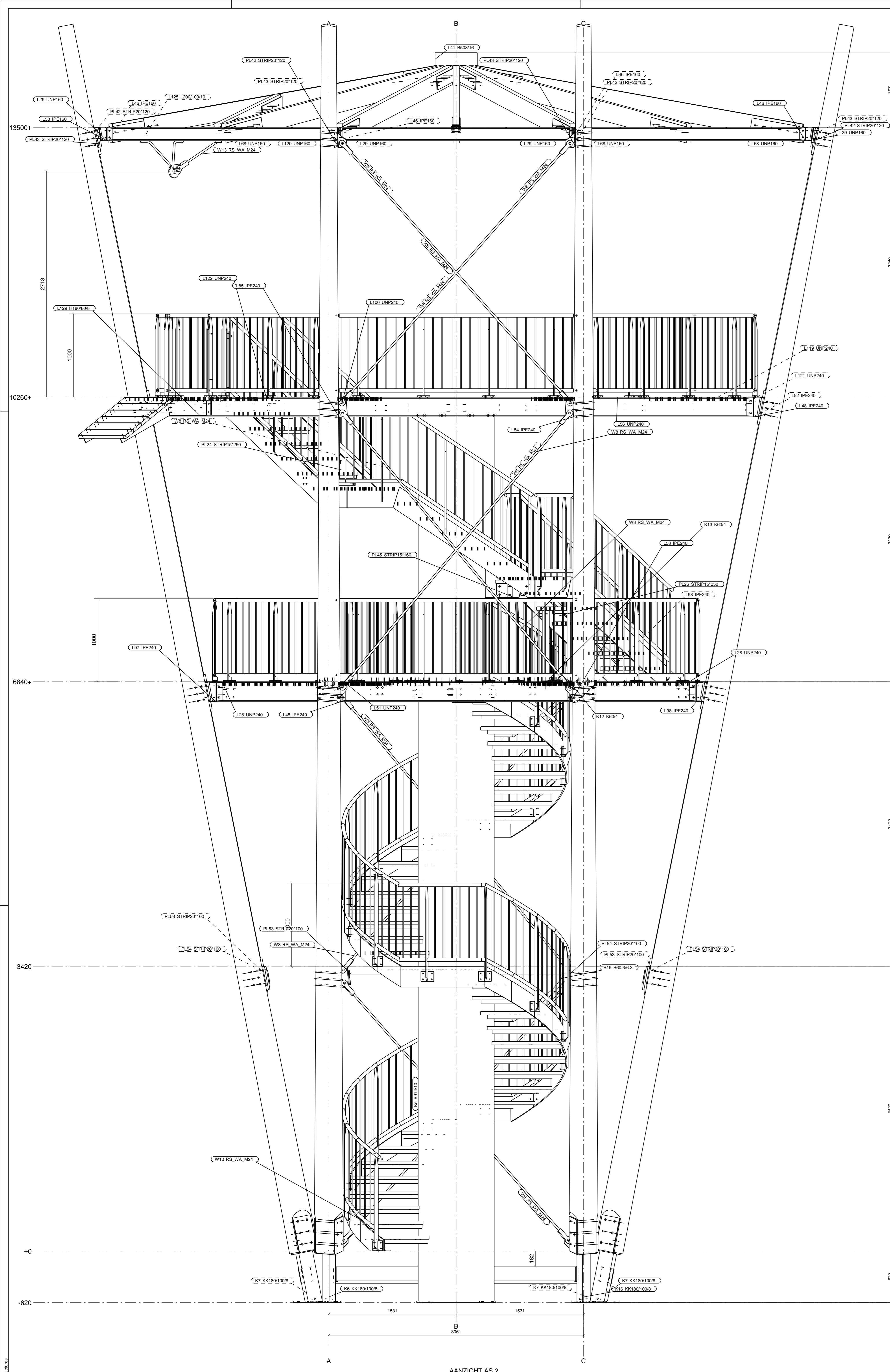
AANZICHT AS 2 1:20
