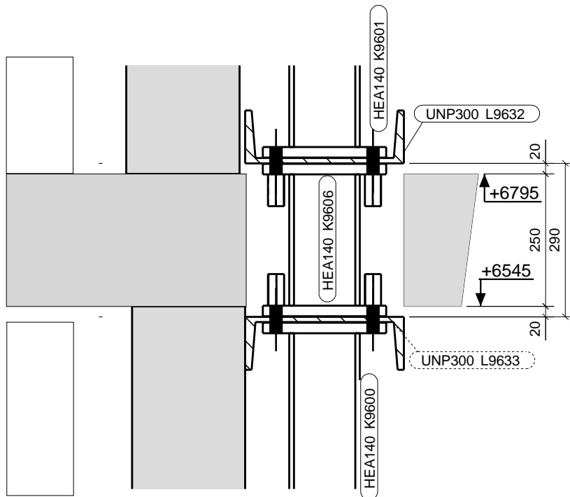
dsn 3.3 - 3.3 , 1:10
