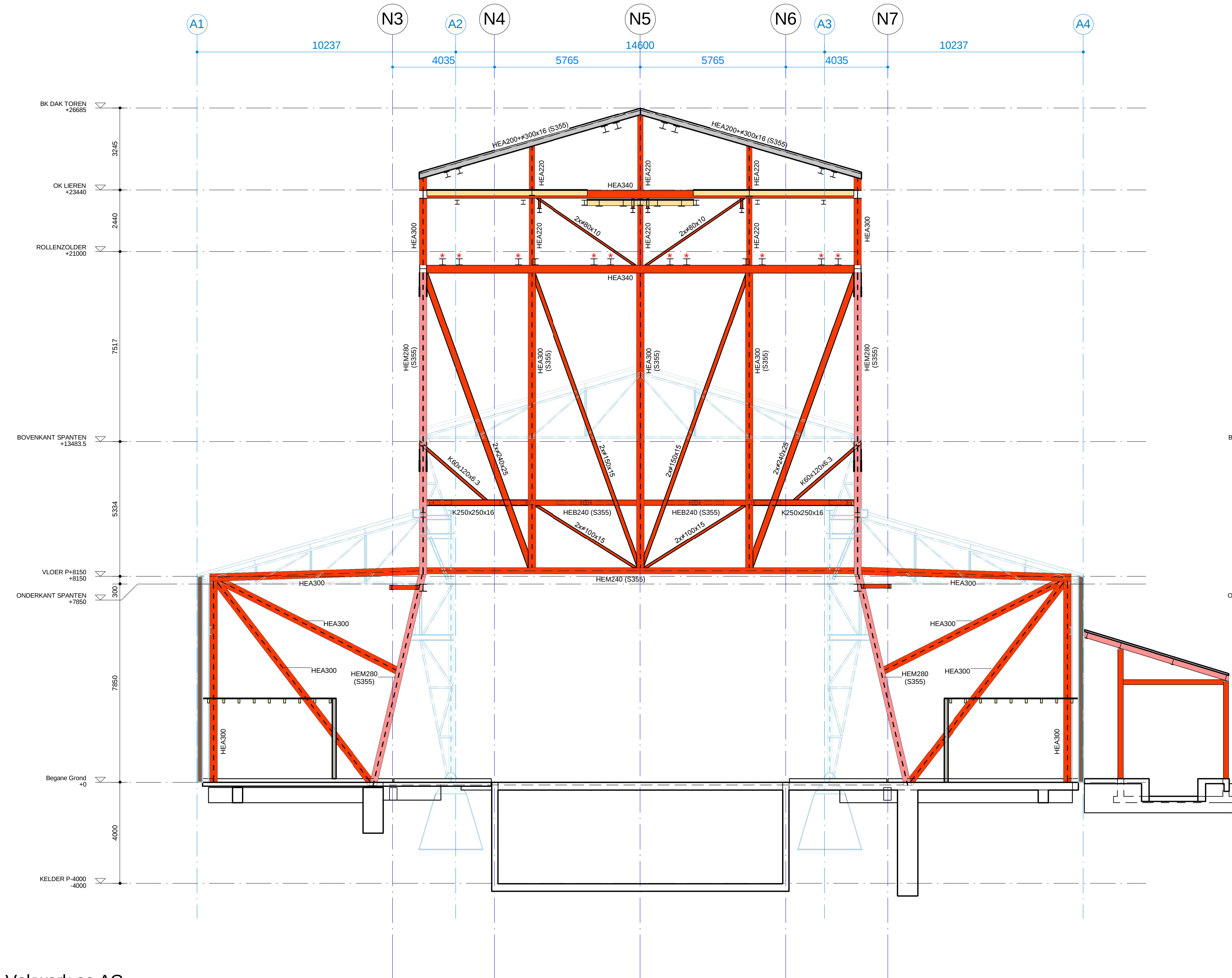
Vakwerk as AG Schaal: 1 : 100
