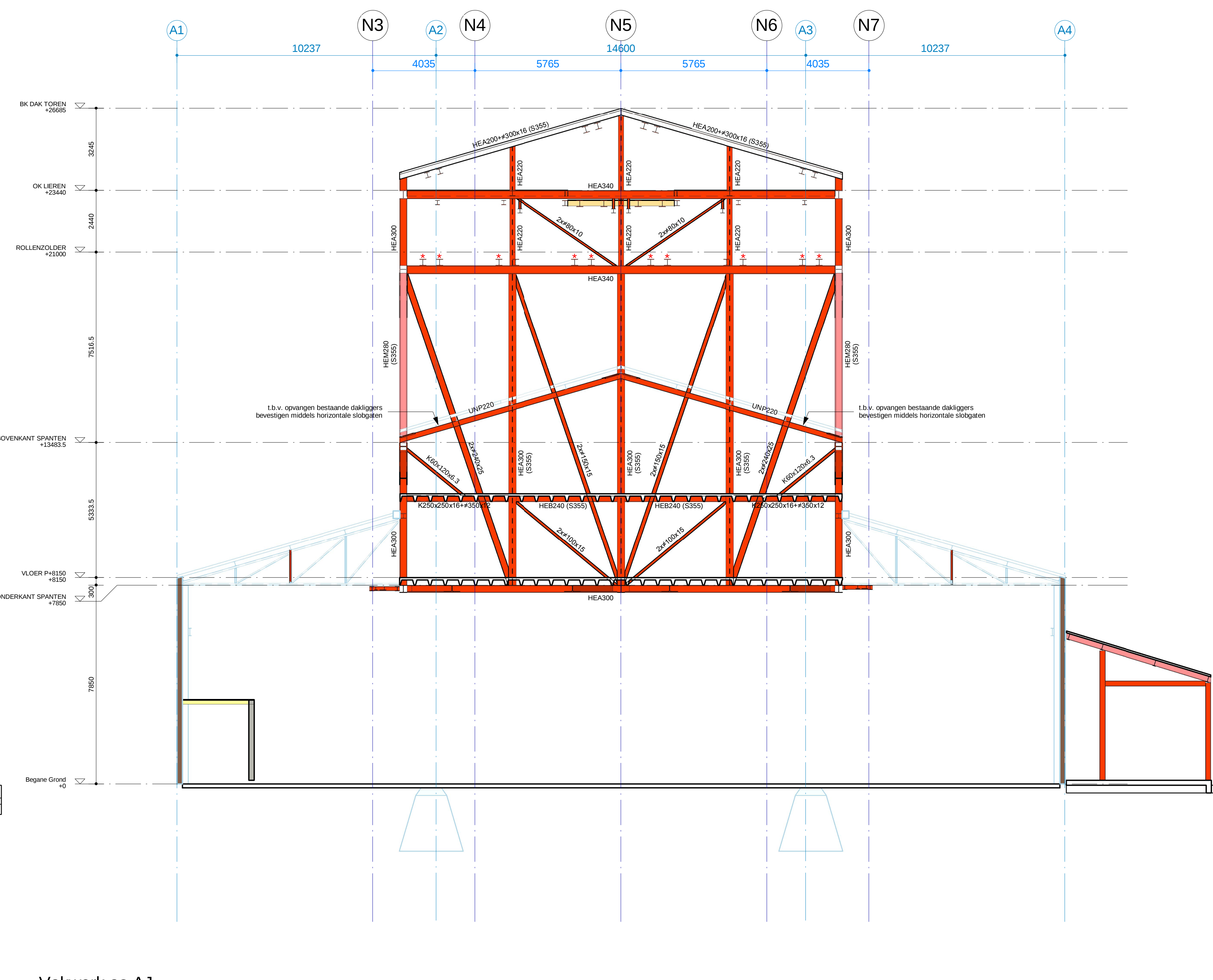
Vakwerk as AJ Schaal: 1 : 100
