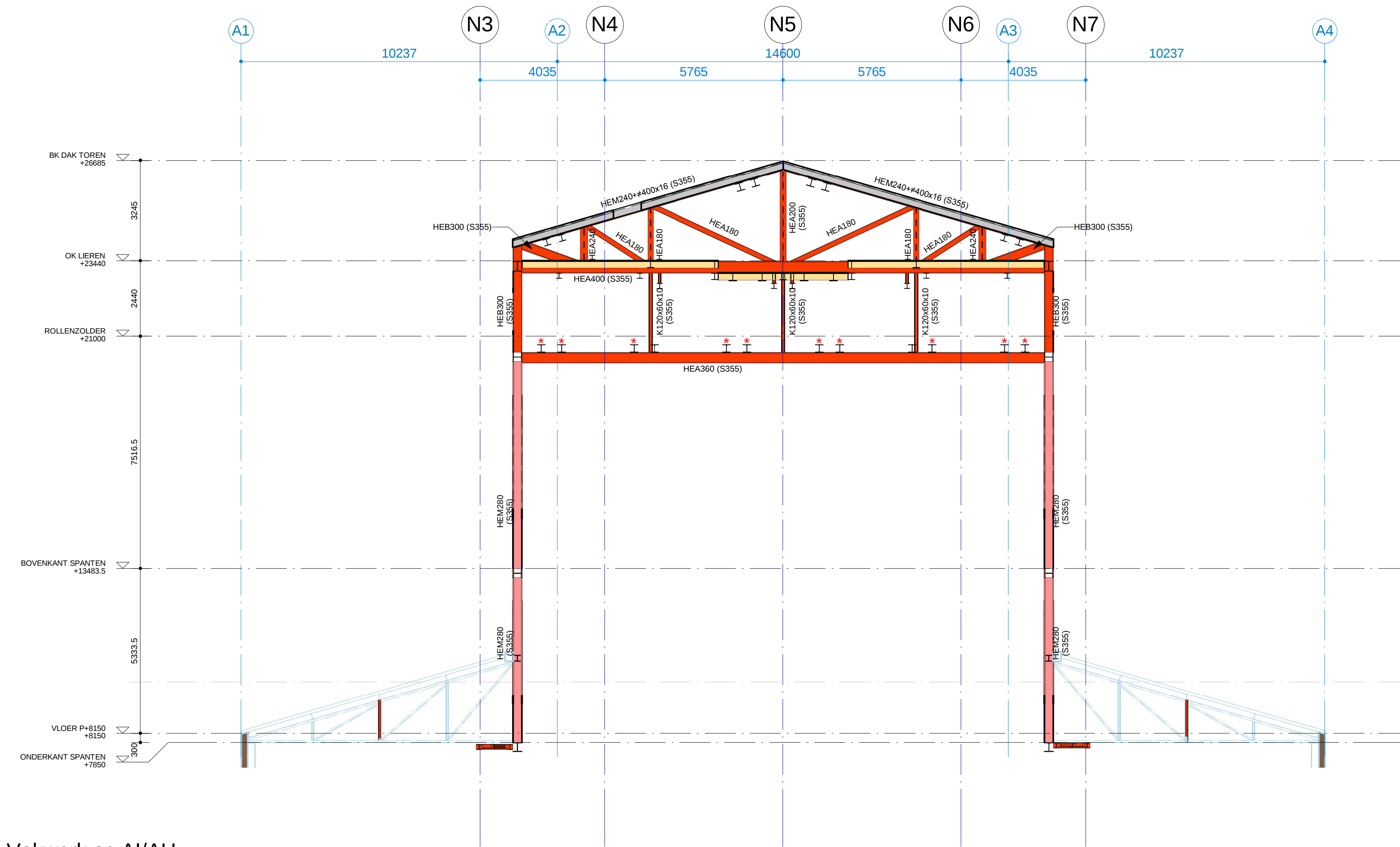
Vakwerk as AI/AH Schaal: 1 : 100
