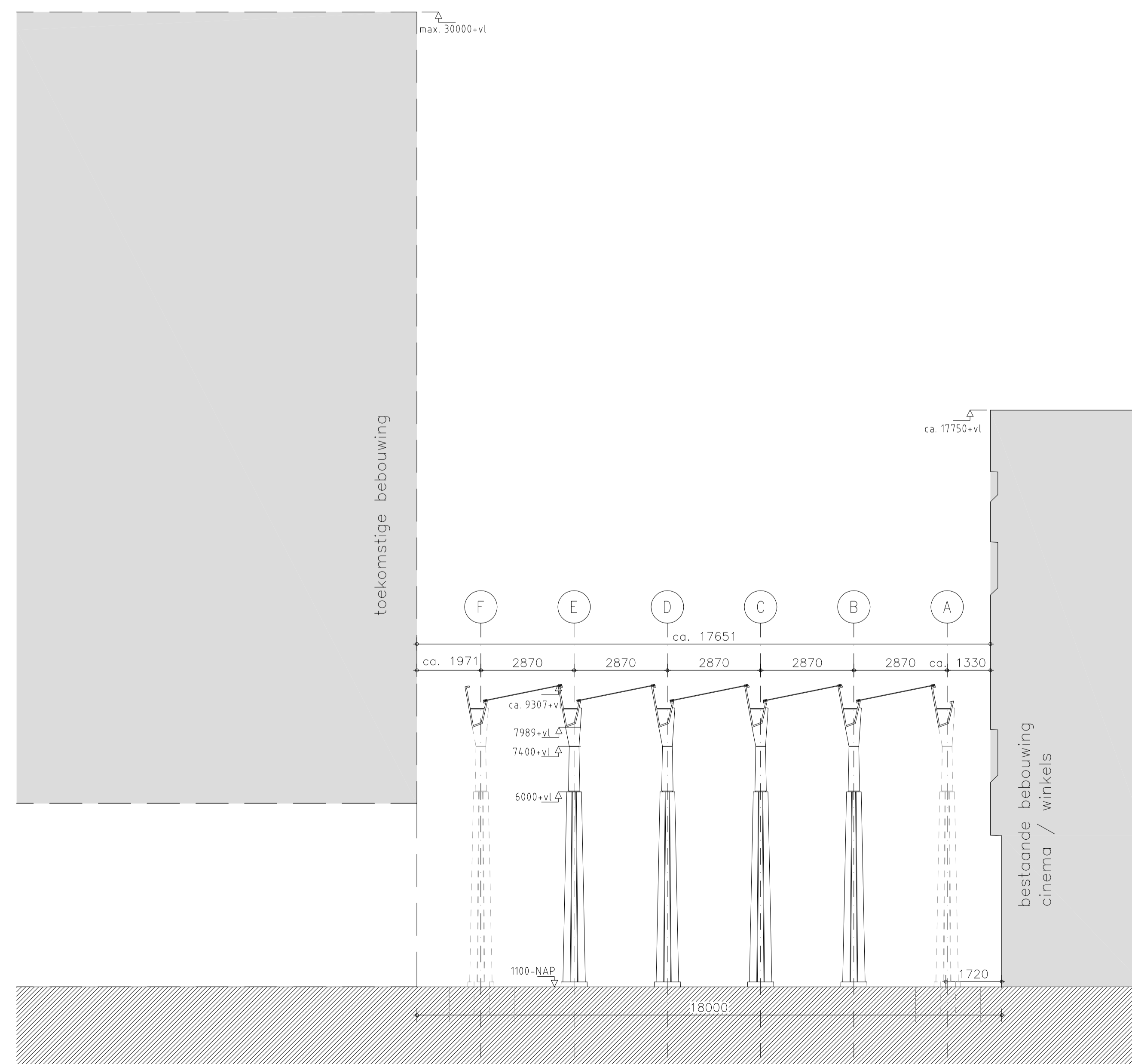
Doorsnede B-B
