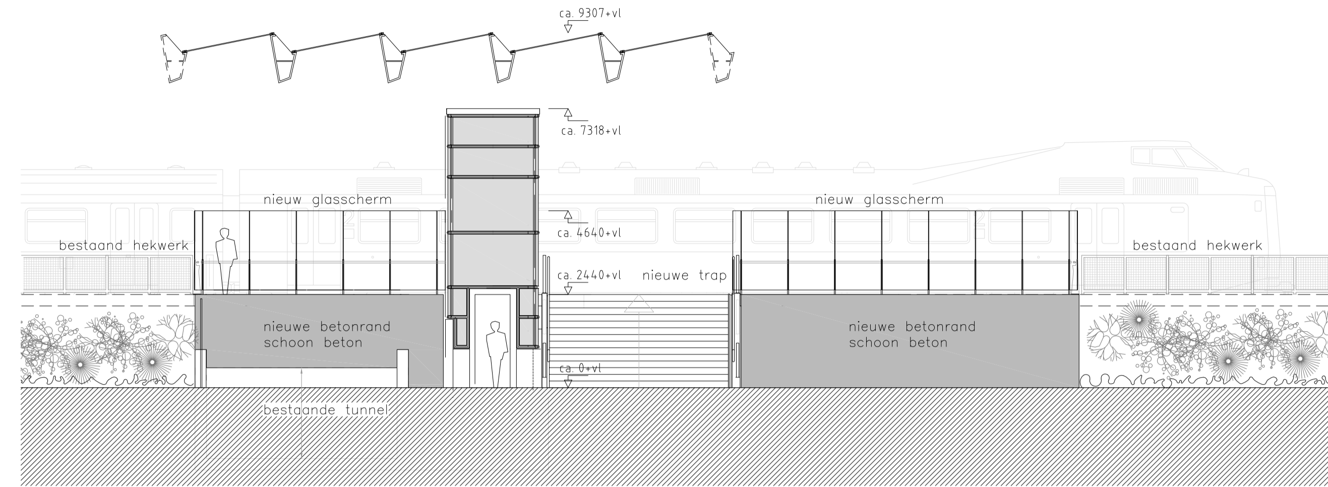
Doorsnede C-C
