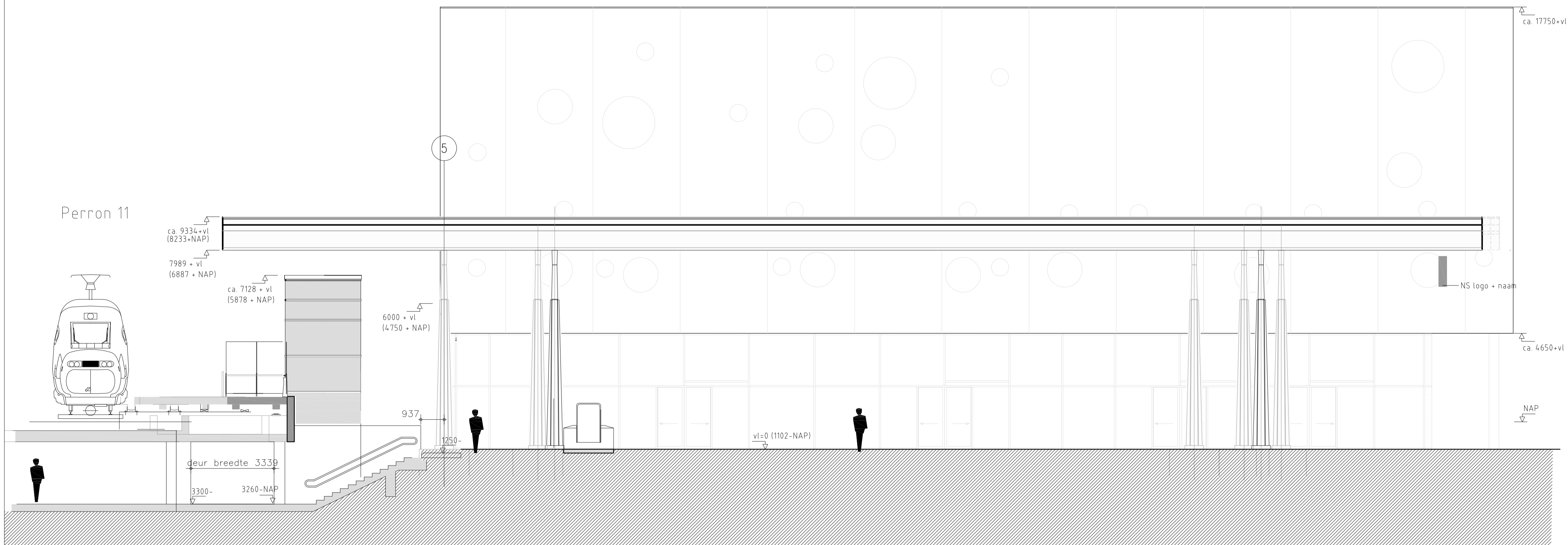
Doorsnede A2-A2
