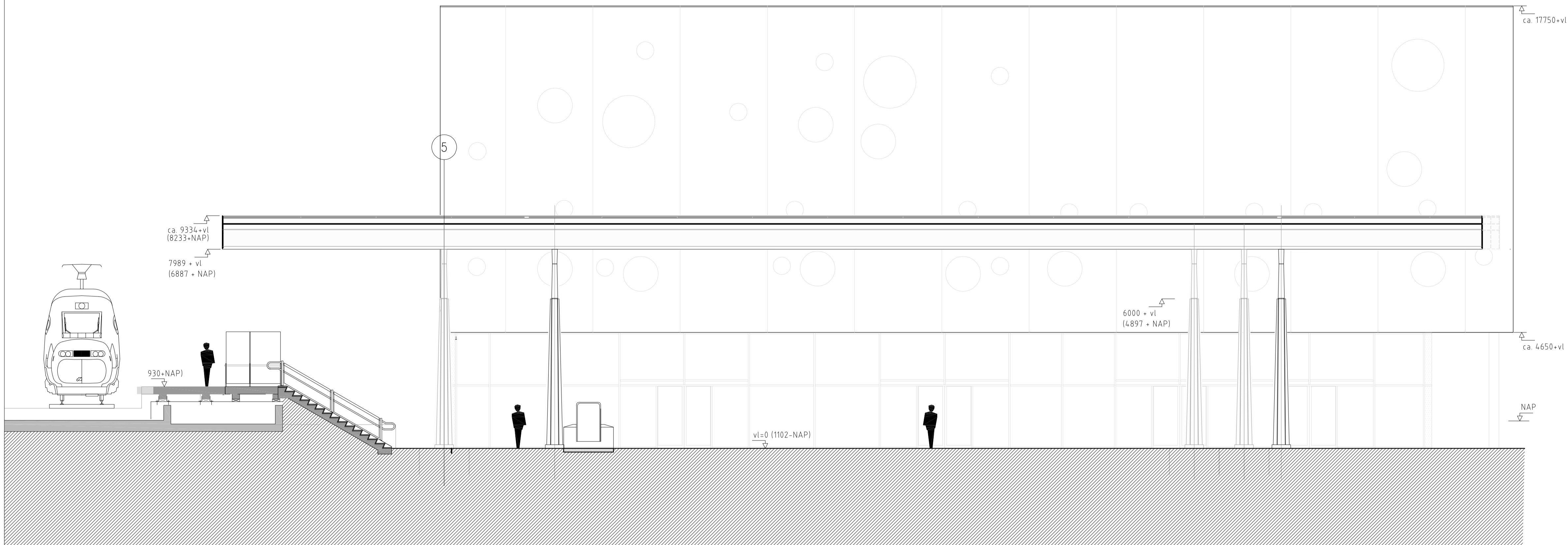
Doorsnede A1-A1
