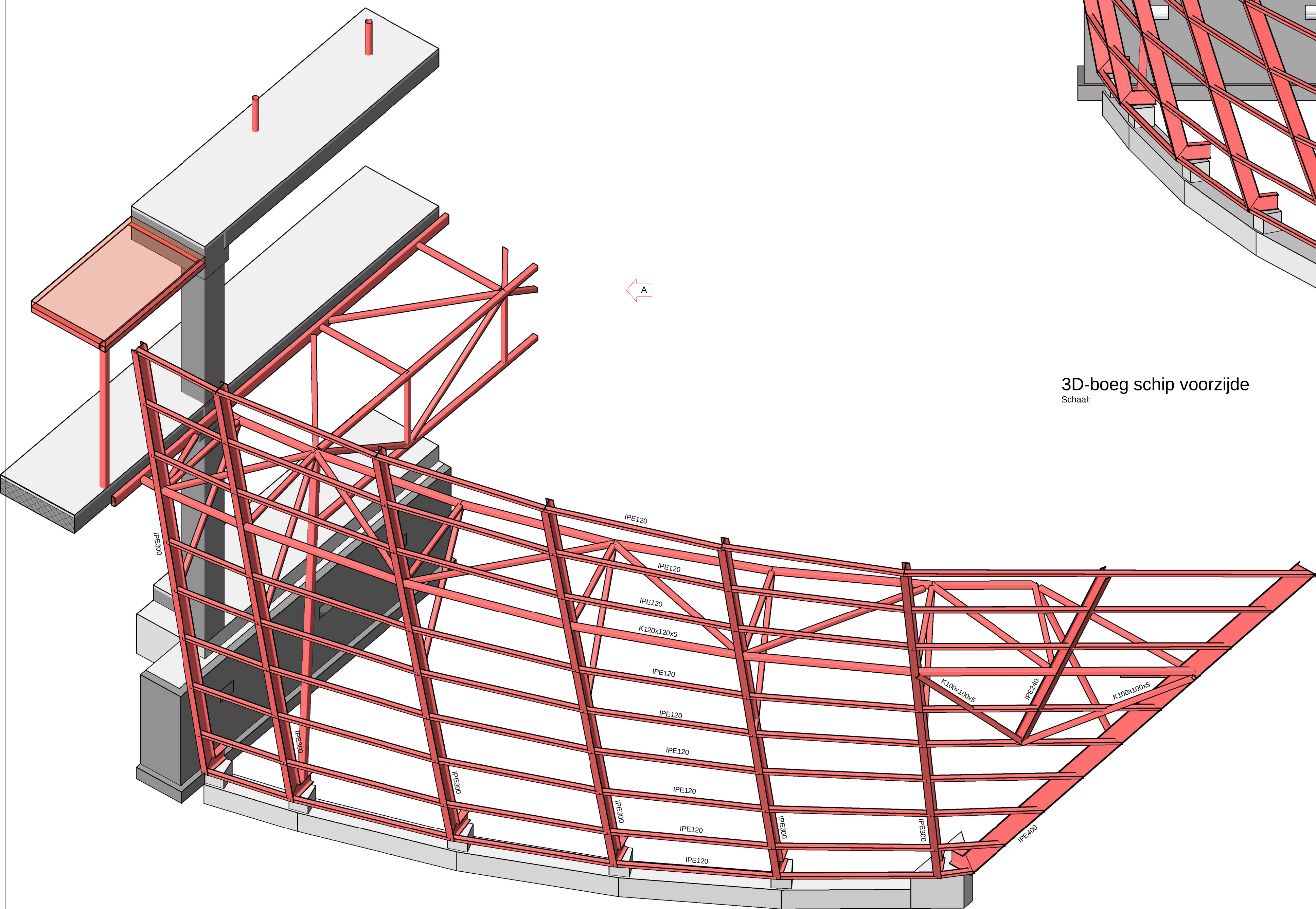
3D-boeg schip links Schaal:
