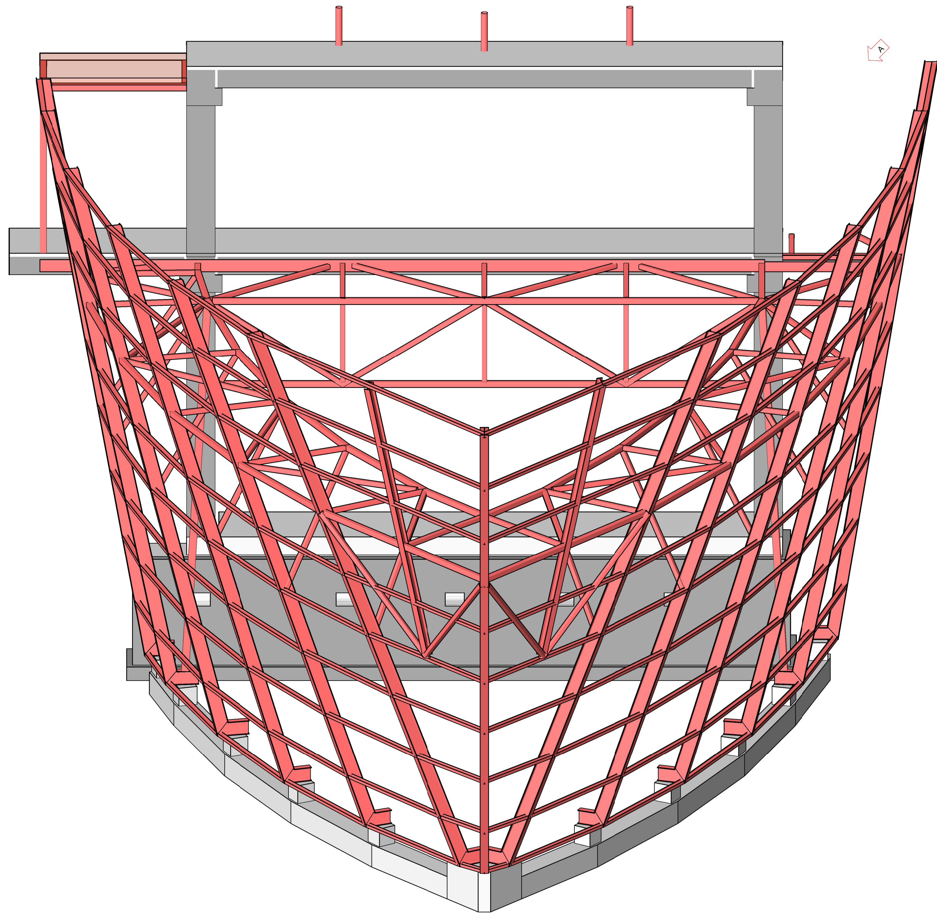
3D-boeg schip voorzijde Schaal:
