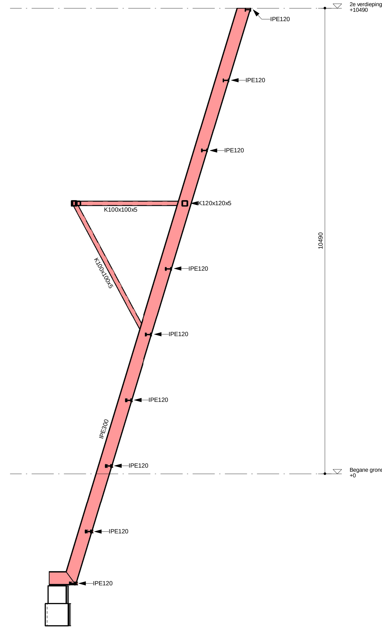
Principe Doorsnede boegspant Schaal: 1 : 50
