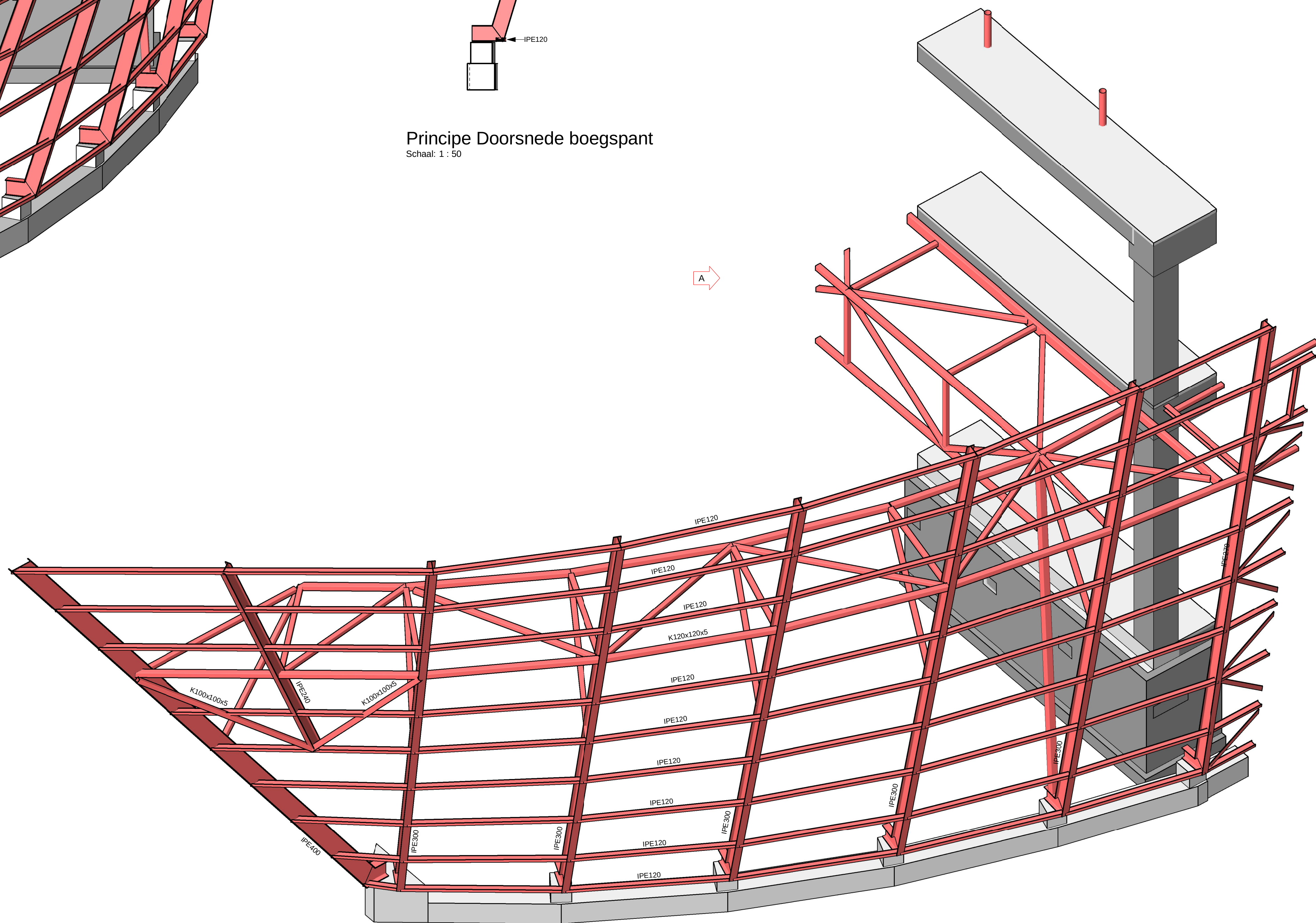
3D-boeg schip rechts Schaal:
