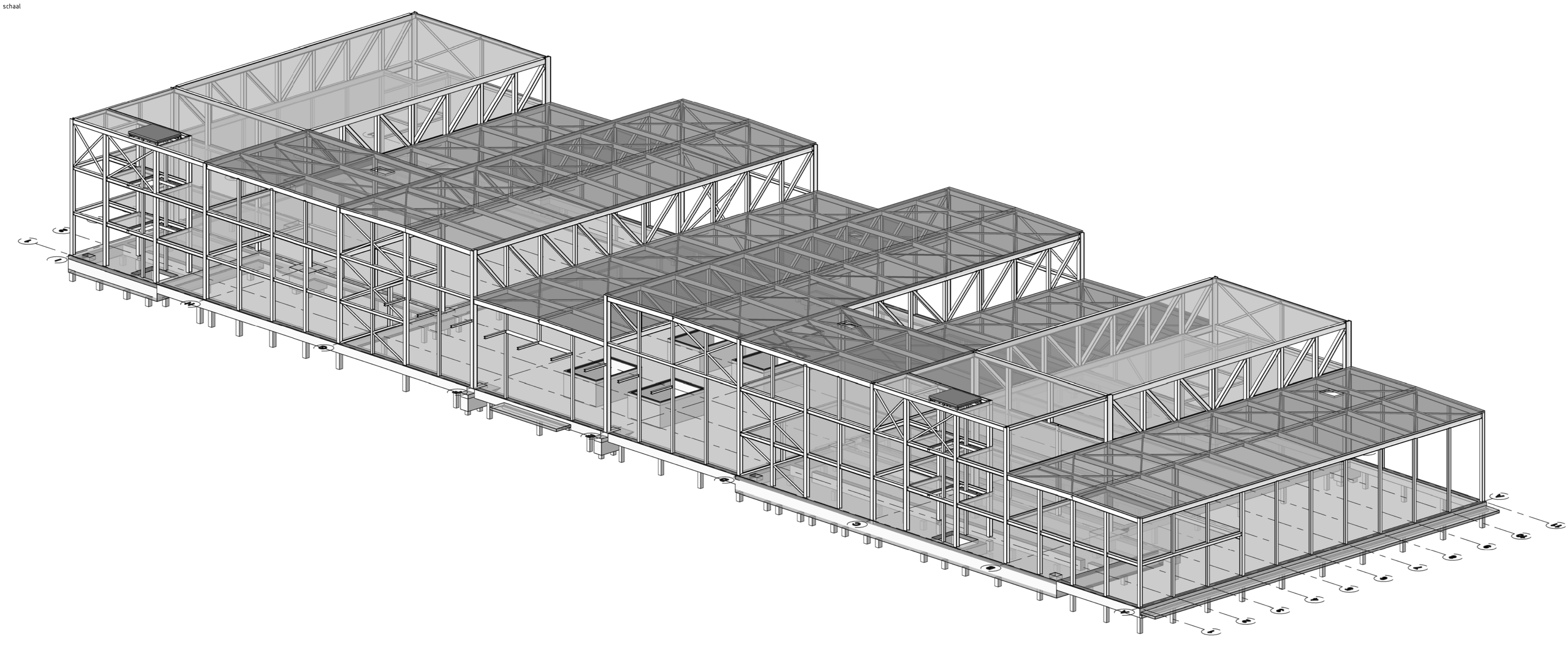
2 3D overzicht staalconstructie as 1 1:100 schaal
