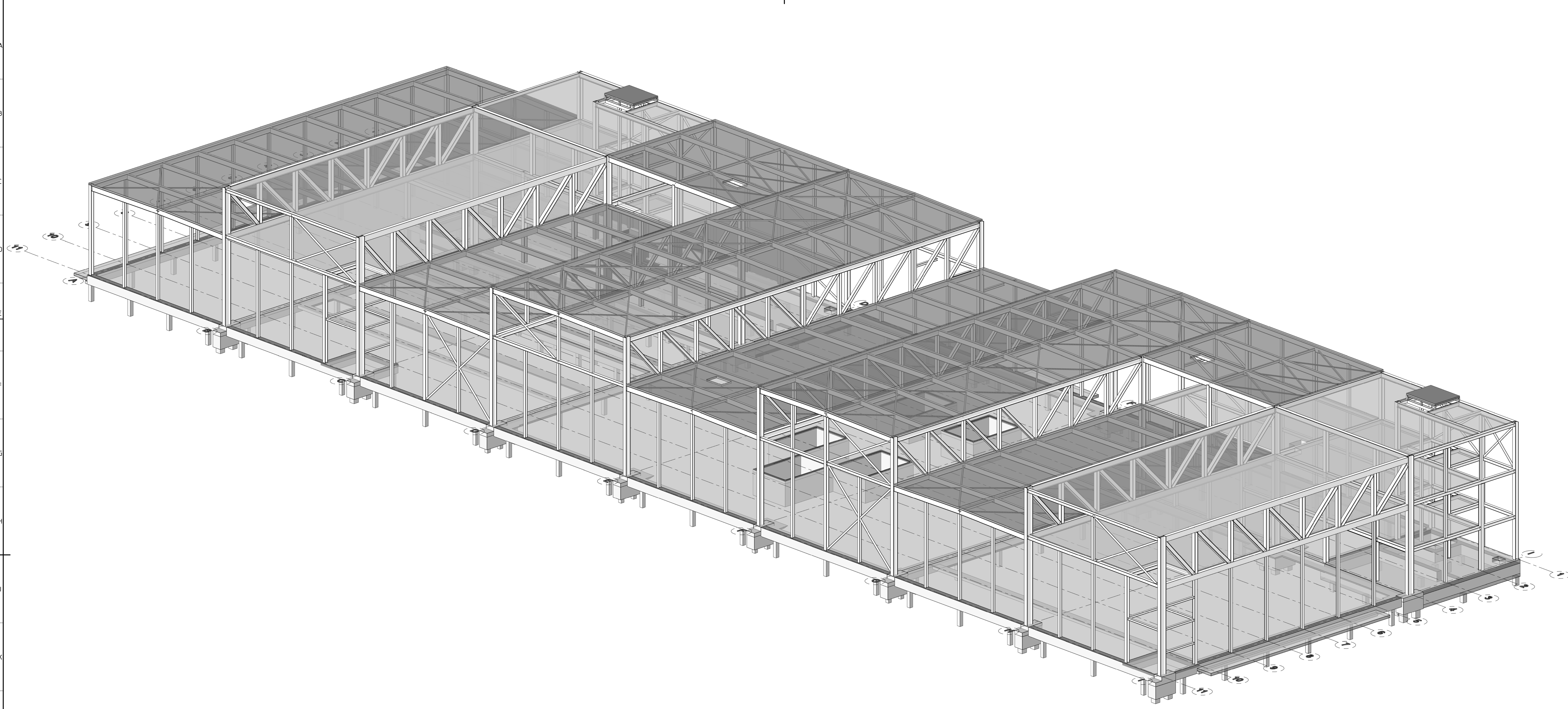
1 3D overzicht staalconstructie 1:100 schaal
