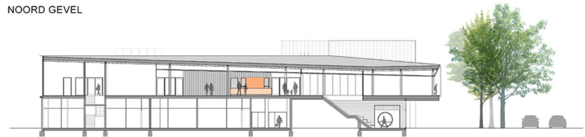
LENGTEDOORSNEDE
