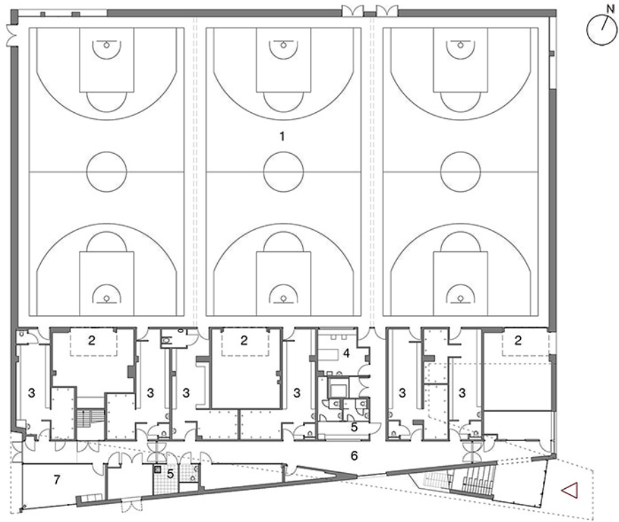
BEGANE GROND
