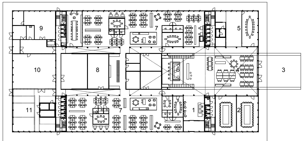
begane grond
