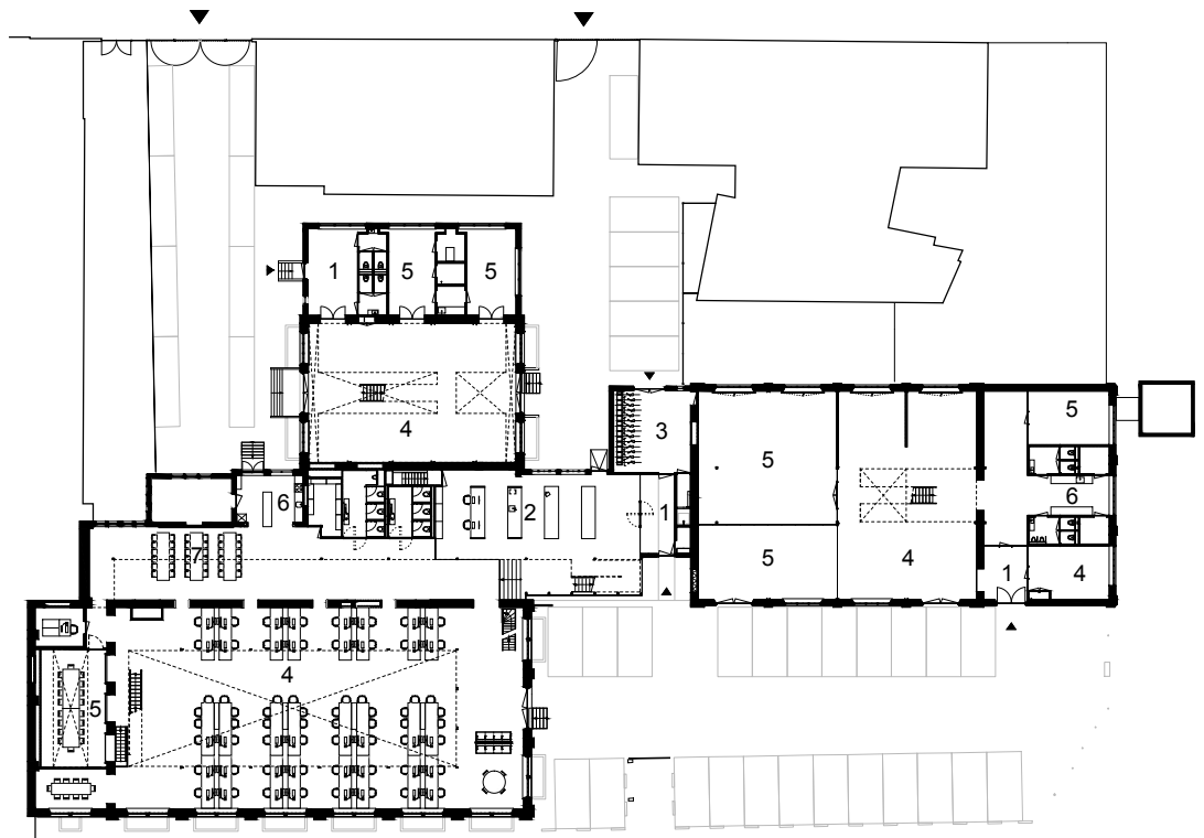
begane grond oorspronkelijke situatie
