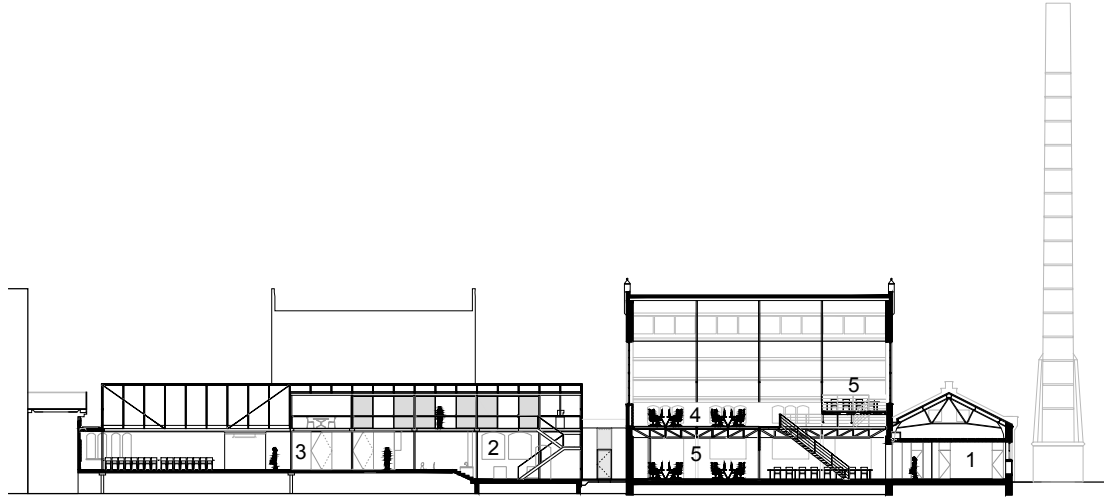
langsdoorsnede nieuwe situatie
