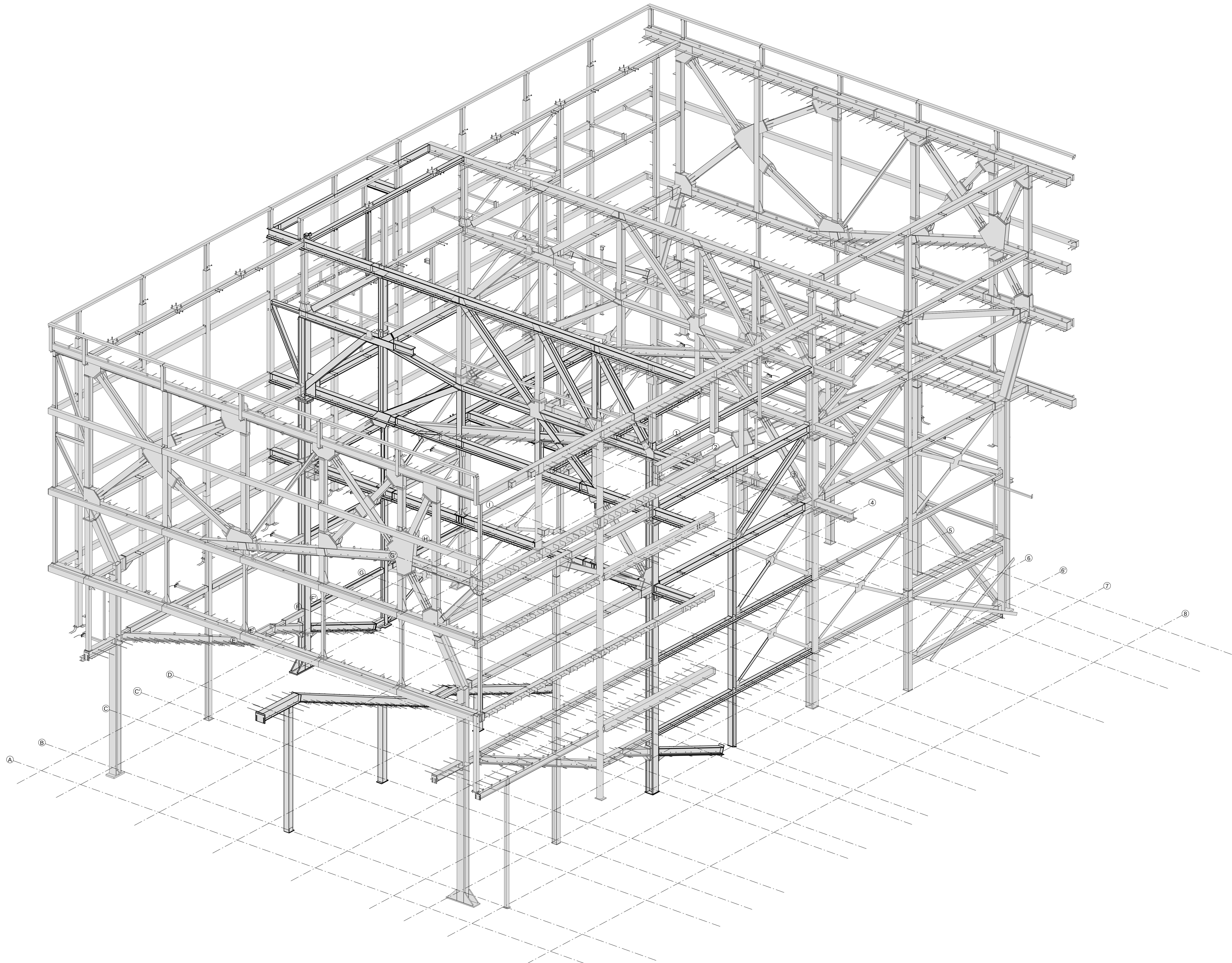
3d Aanzicht 1:60
