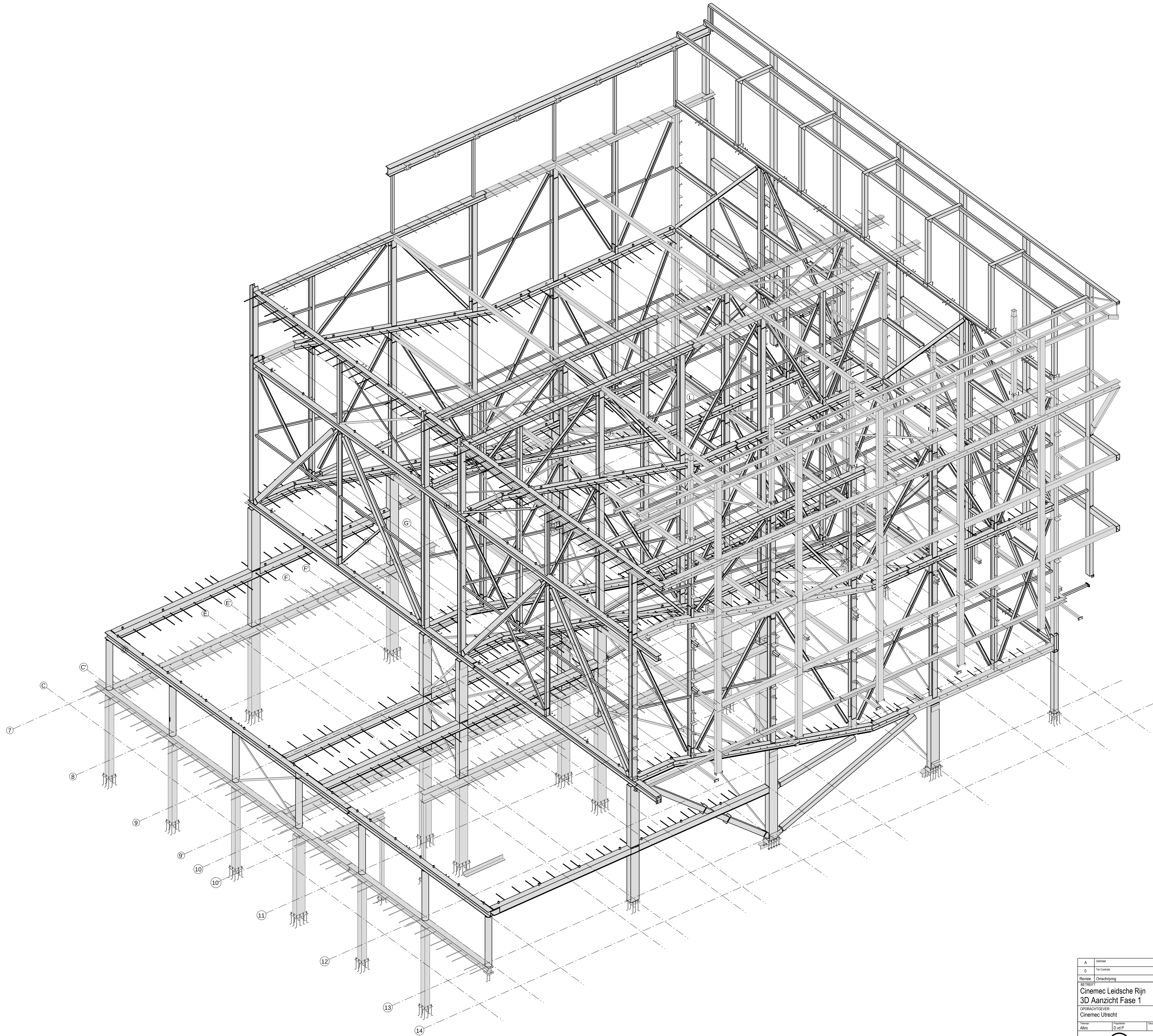
3d Aanzicht 1:60
