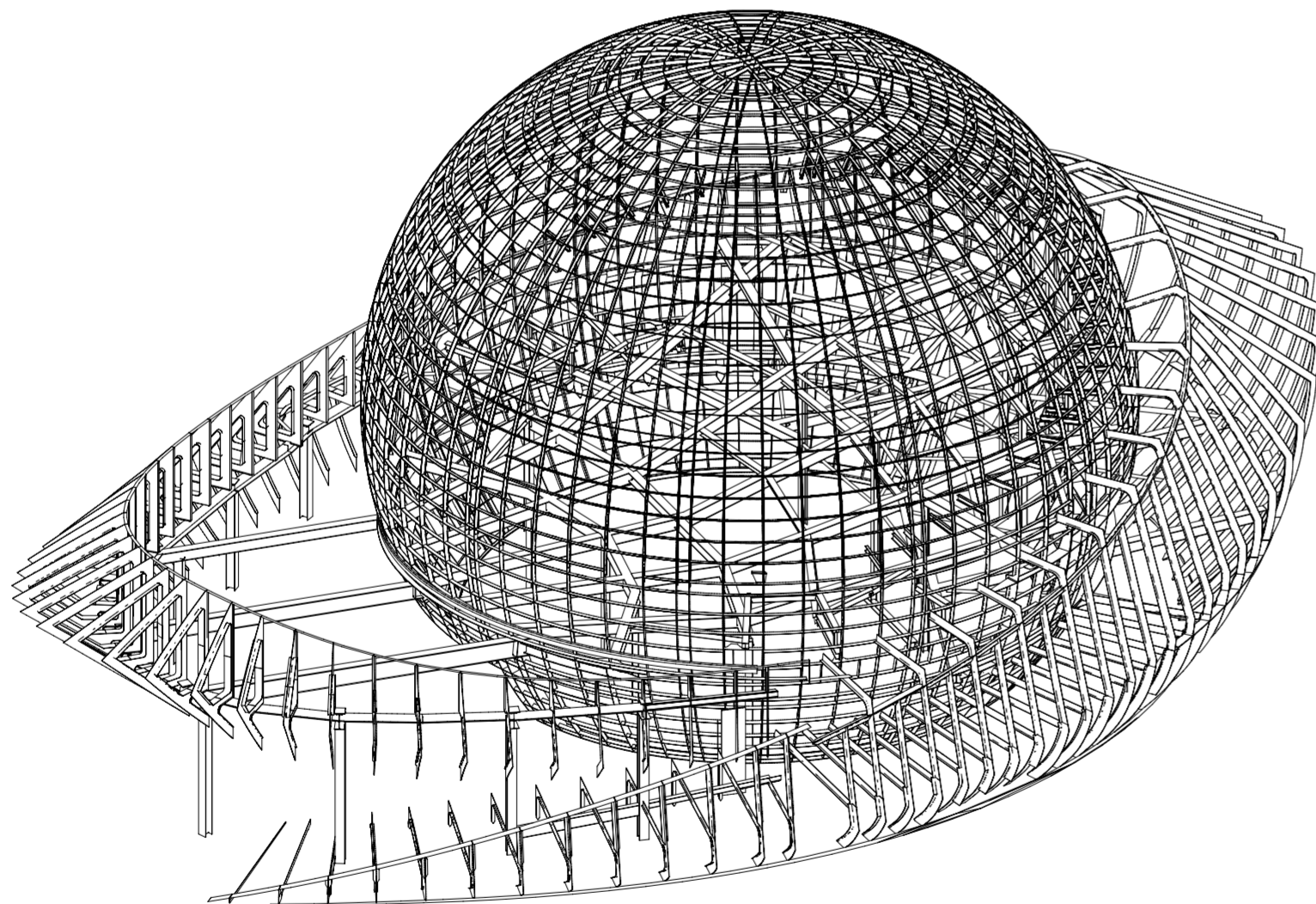
STAALCONSTRUCTIE TOTAAL
