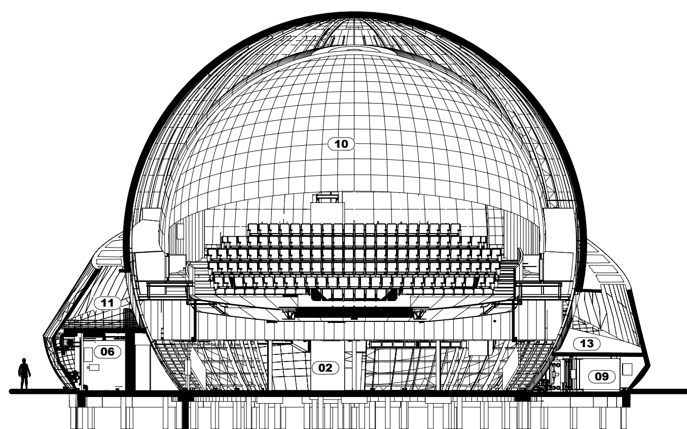
DWARSDOORSNEDE
