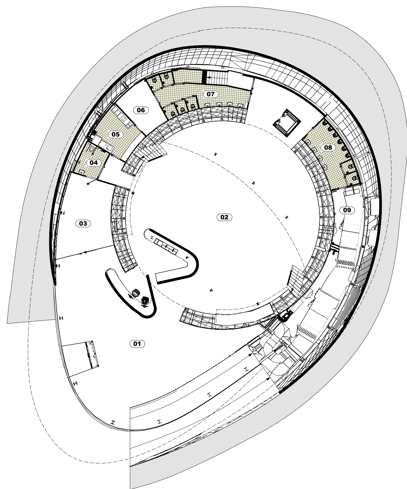
BEGANE GROND
