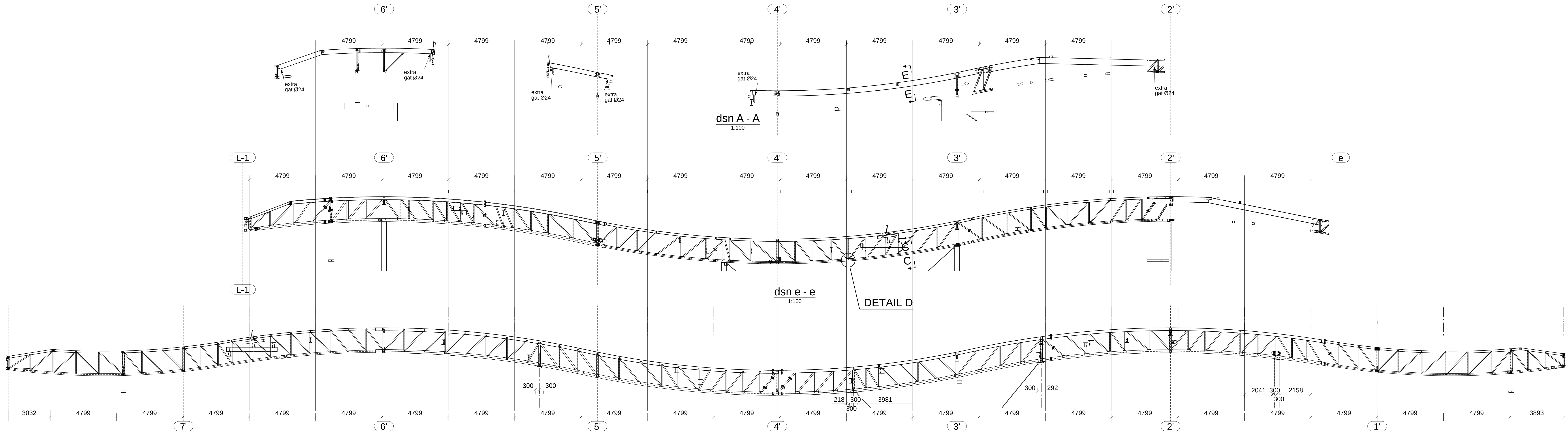
dsn C - C , 1:100
