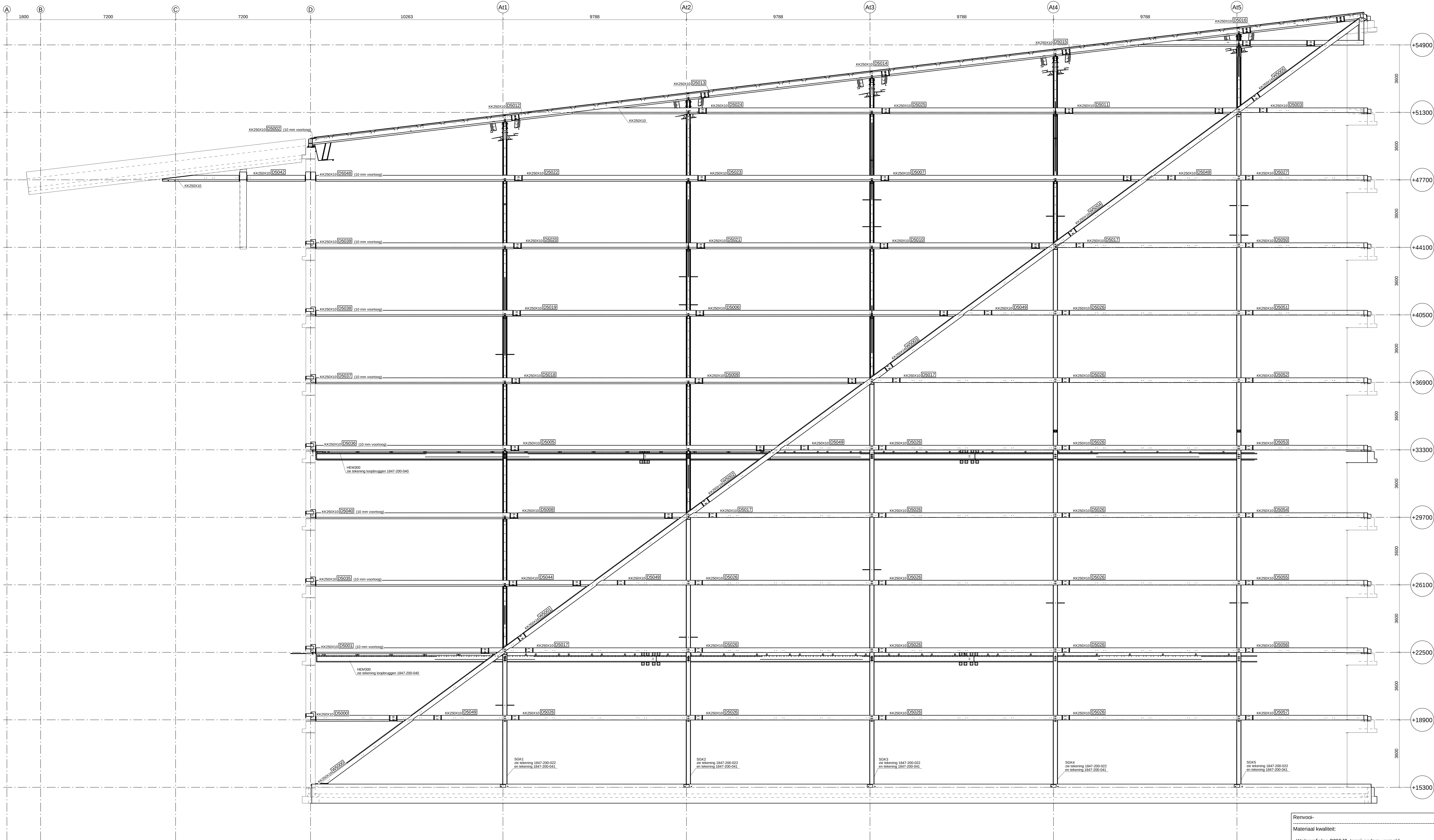
Aanzicht Noordgevel (loodrecht op kolommen) Schaal 1:70
