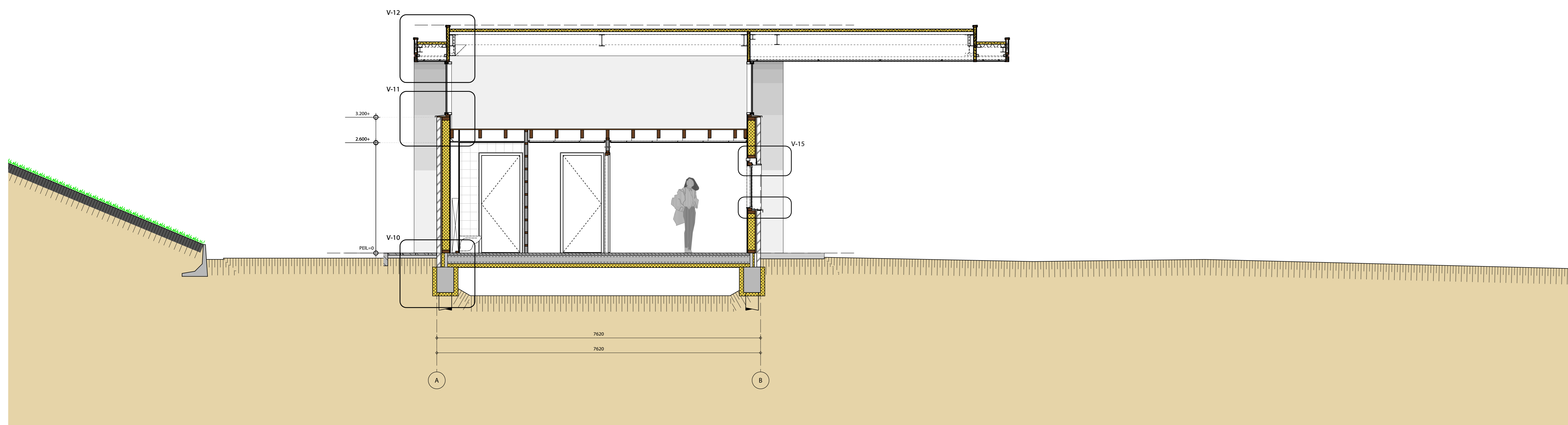
Doorsnede B-B
