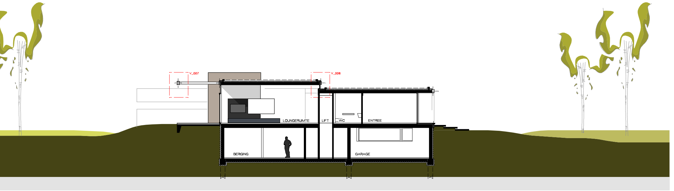
DOORSNEDE A-A'
