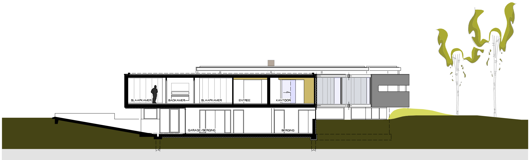
DOORSNEDE B-B'
