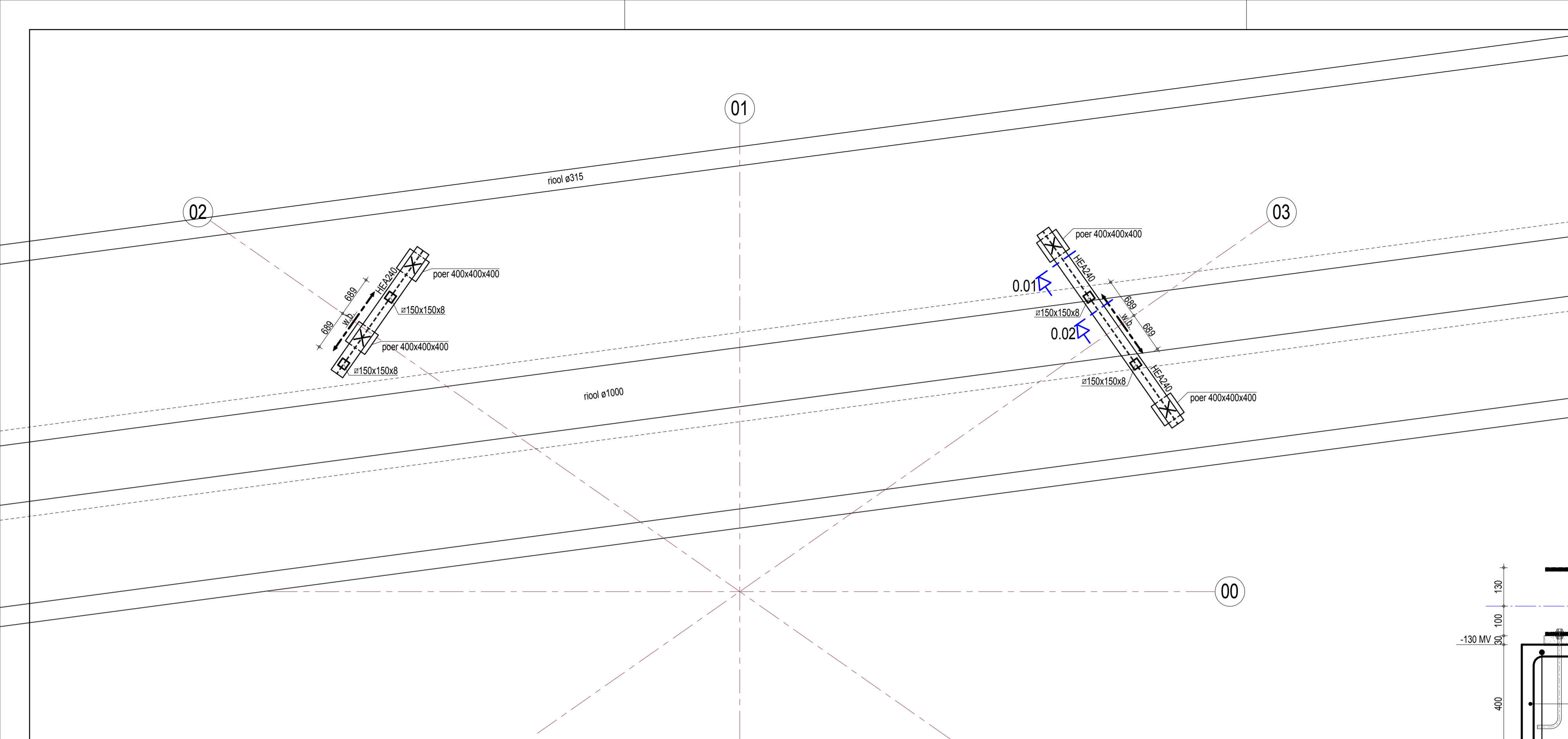
Fundering 1 : 50
