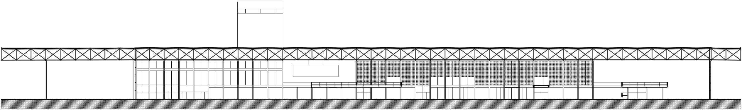
Doorsnede A
