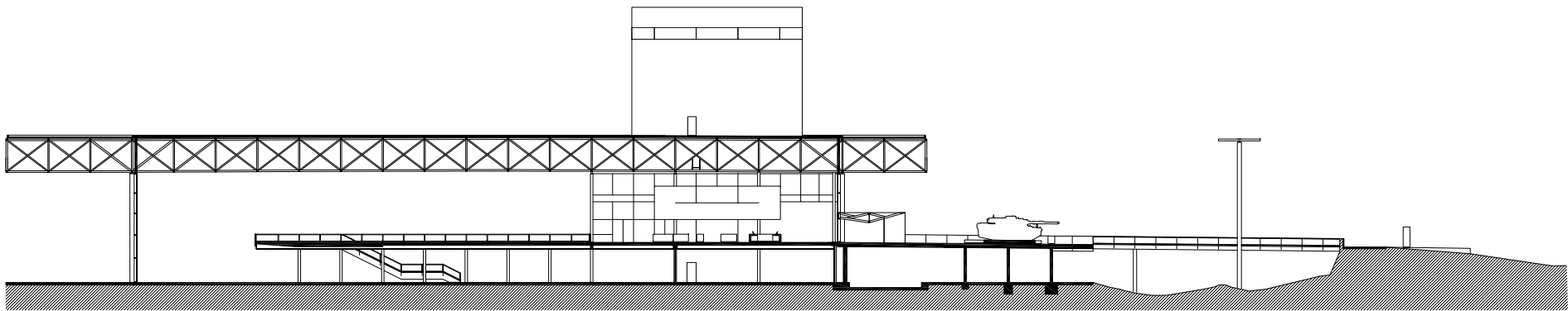
Doorsnede D
