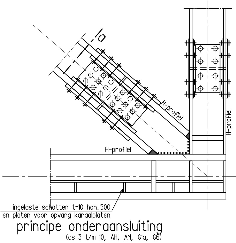
principe bovenaansluiting (as 11 t/m 15b)
