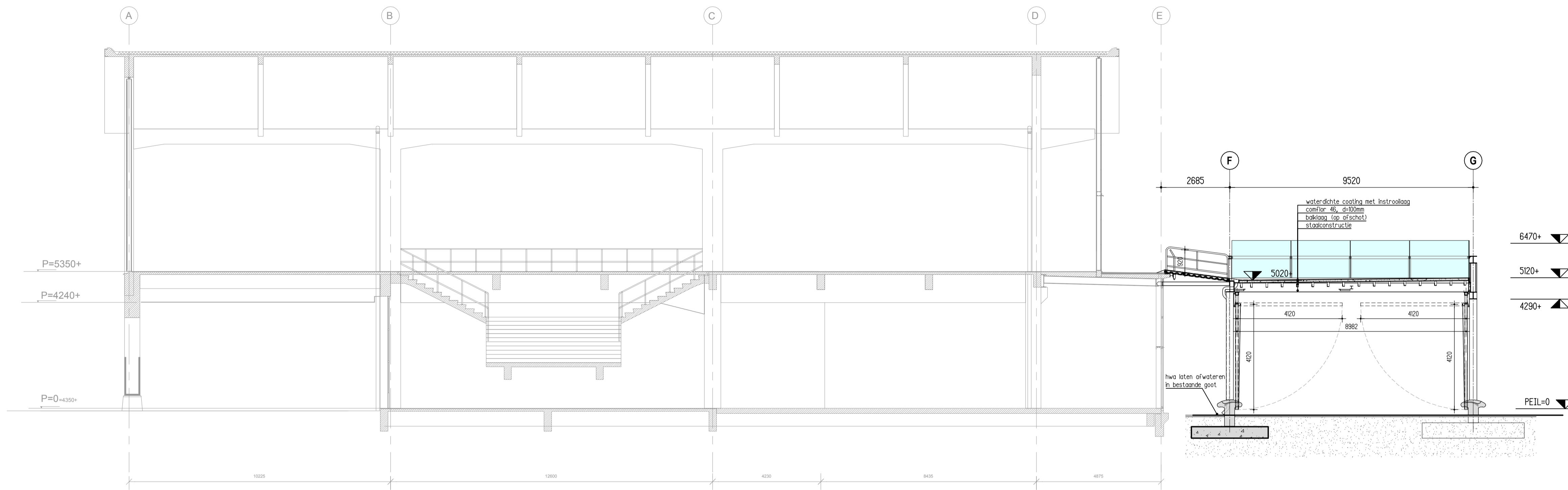
DOORSNEDE A-A nieuwe situatie
