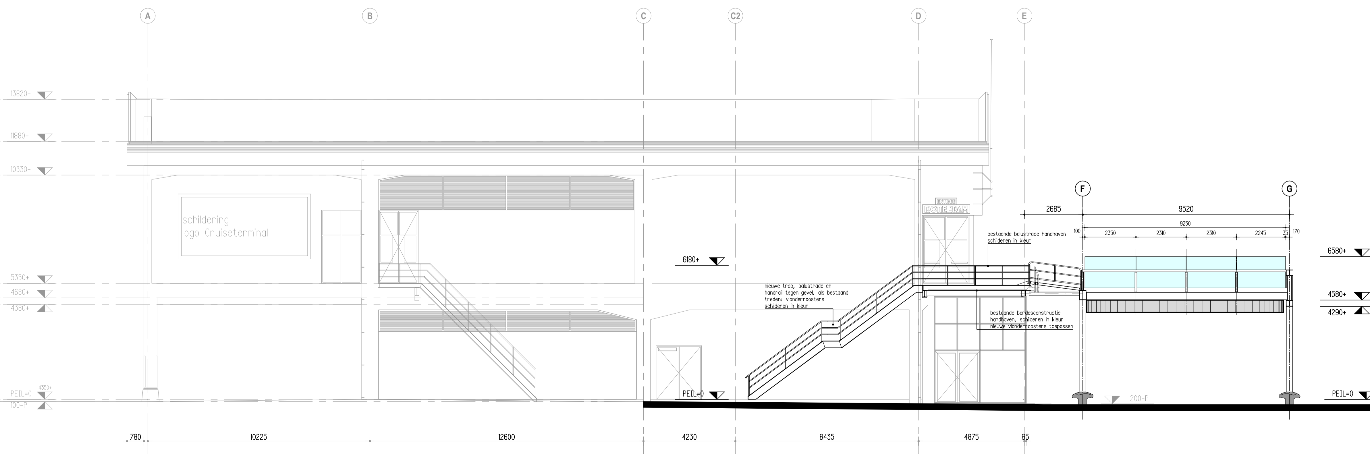
OOSTEGEVEL nieuwe situatie
