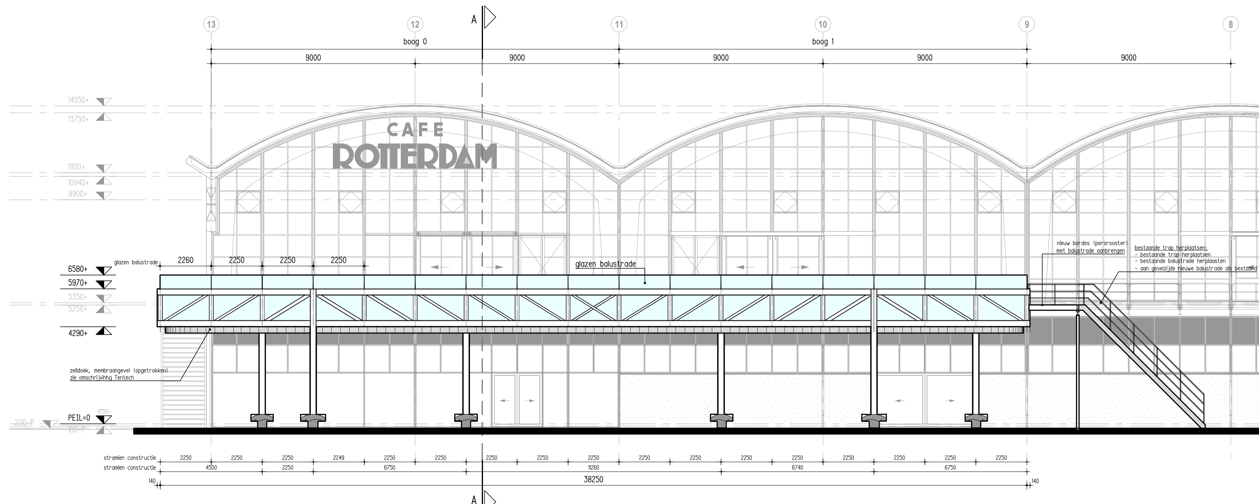
ACHTERGEVEL WILHELMINAKADE 699 (rivierzijde) Bagage-ruimte niet in gebruik, zeildoek opgeborgen.
