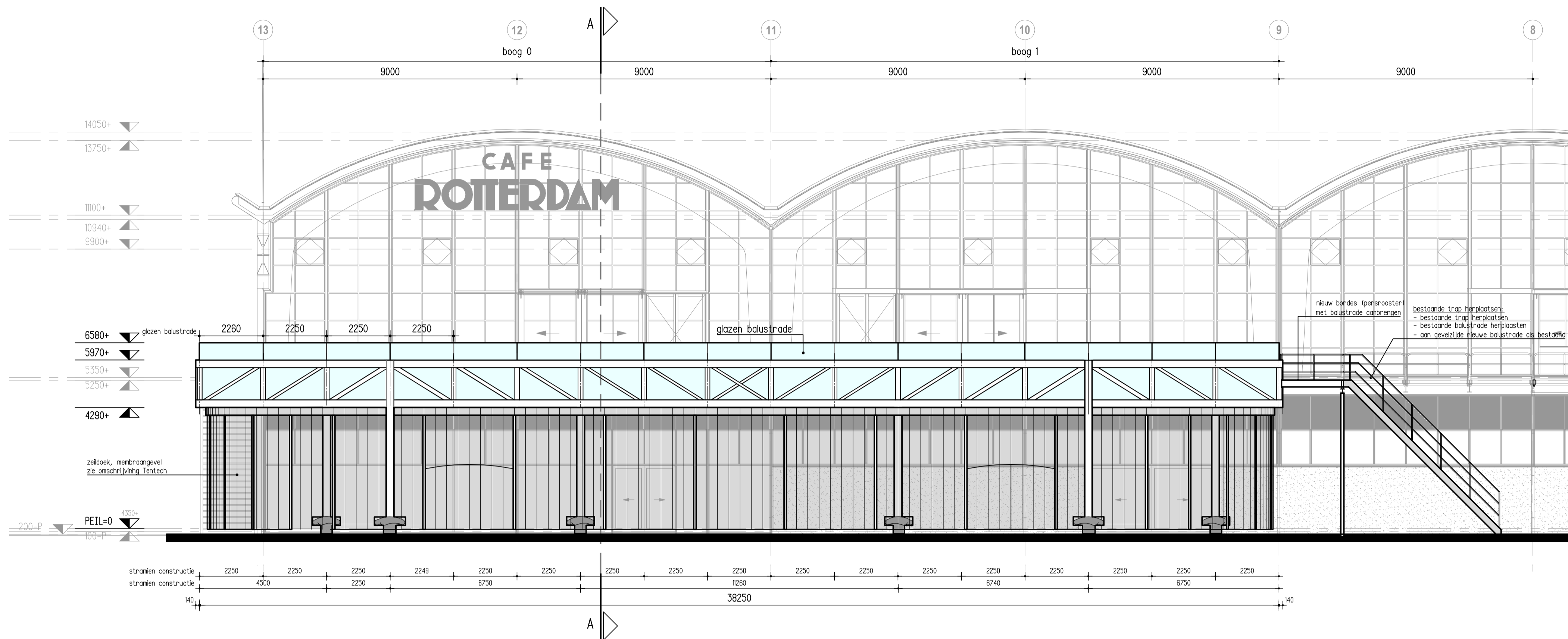
ACHTERGEVEL WILHELMINAKADE 699 (rivierzijde) Bagage-ruimte in gebruik, zeildoek gevel.
