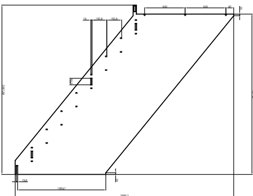
SZ25 20mm - Ansicht 1x
