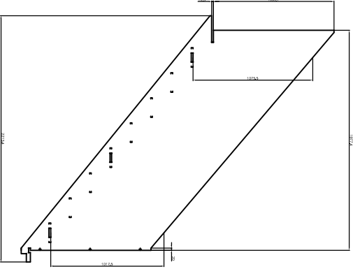
SZ25 20mm - Ansicht 1x
