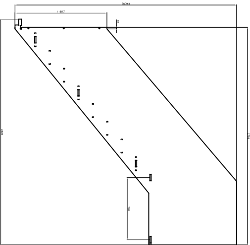
SZ25 20mm - Ansicht 1x
