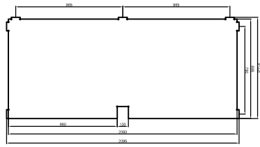
SZ25 15mm - Ansicht 1x
