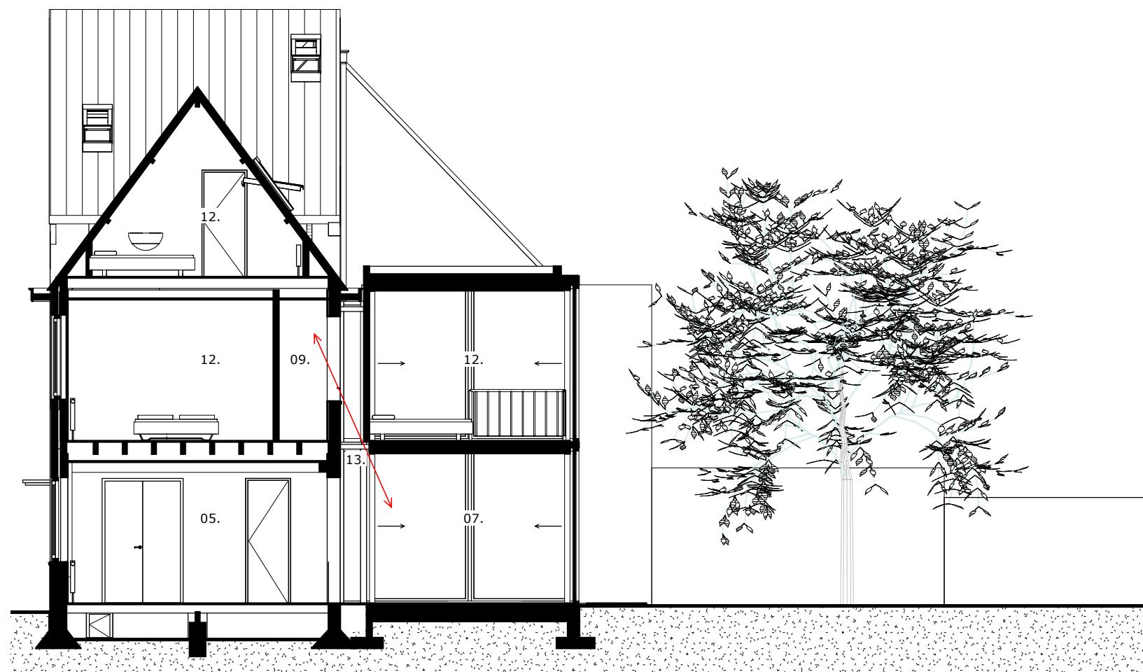
Dwarsdoorsnede Nieuw
