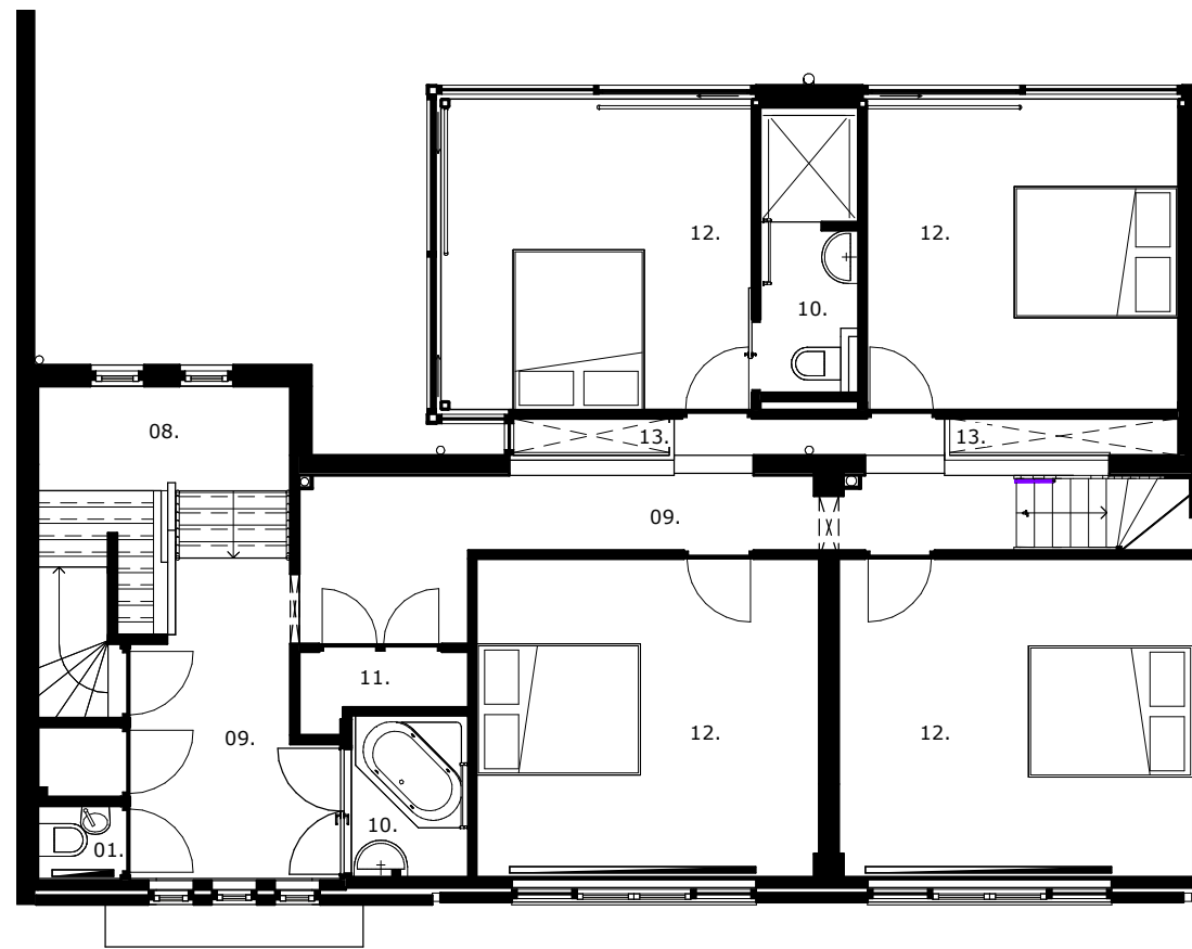
1e Verdieping Nieuw
