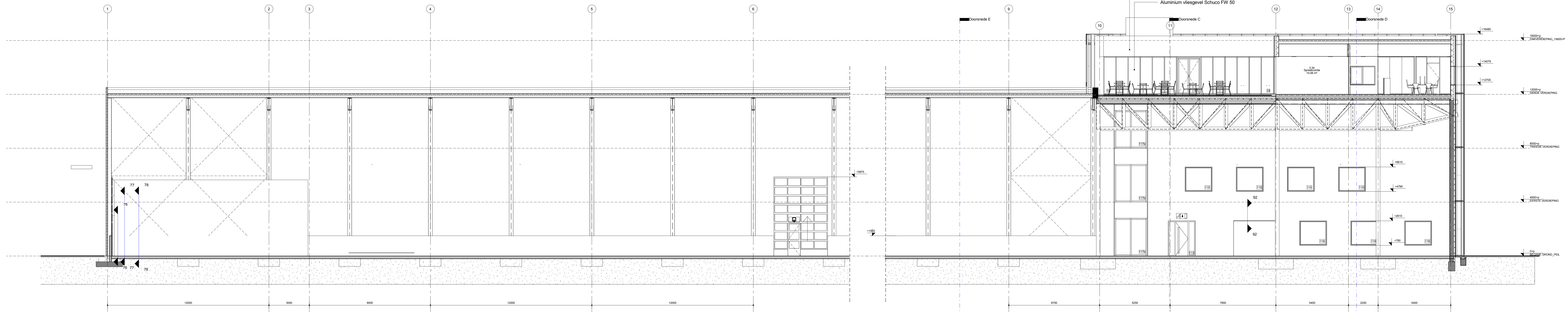
DOORSNEDE B-1
