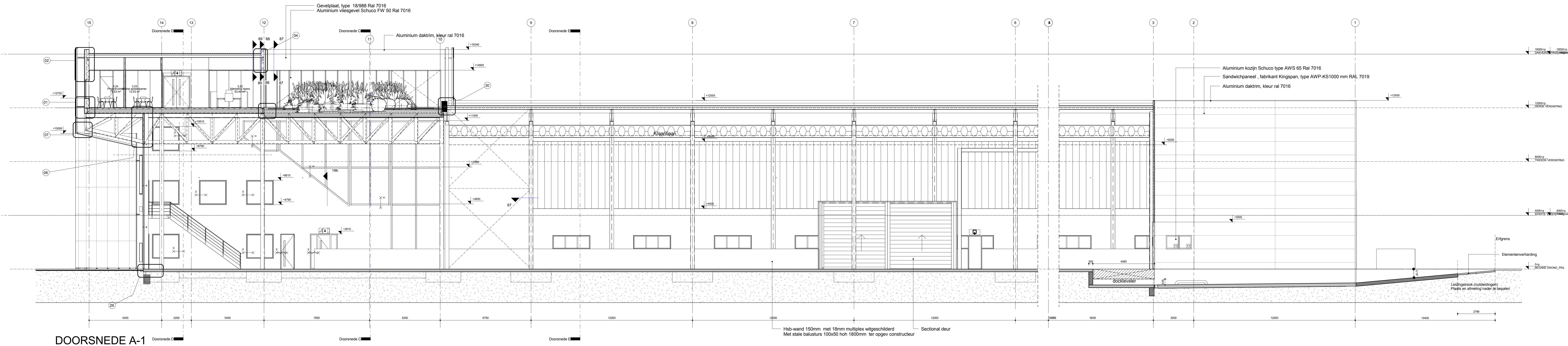
DOORSNEDE A-1
