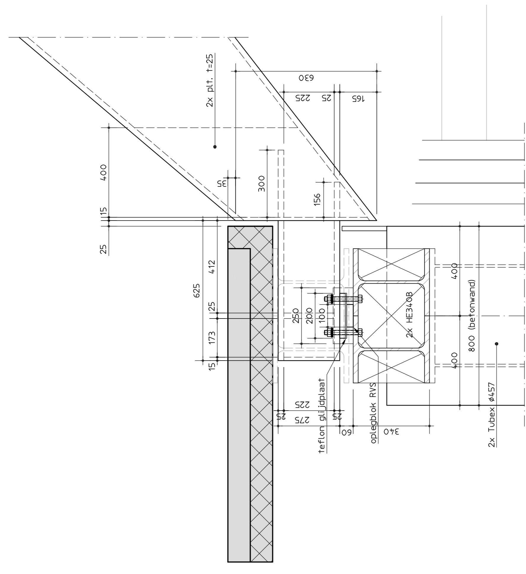
Detail 5 (glijdoplegging)
