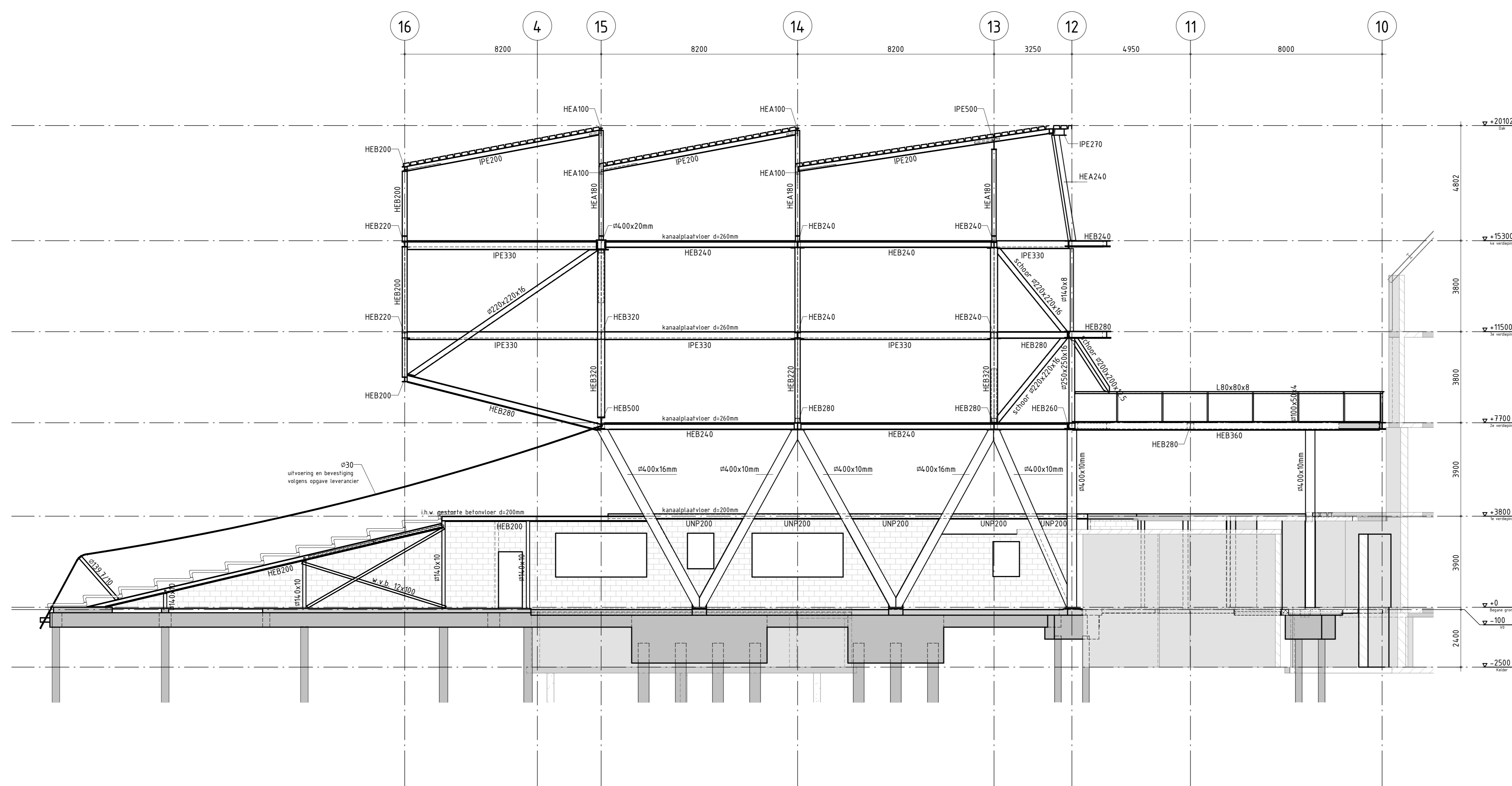
Drsn: J-J 1 : 100
