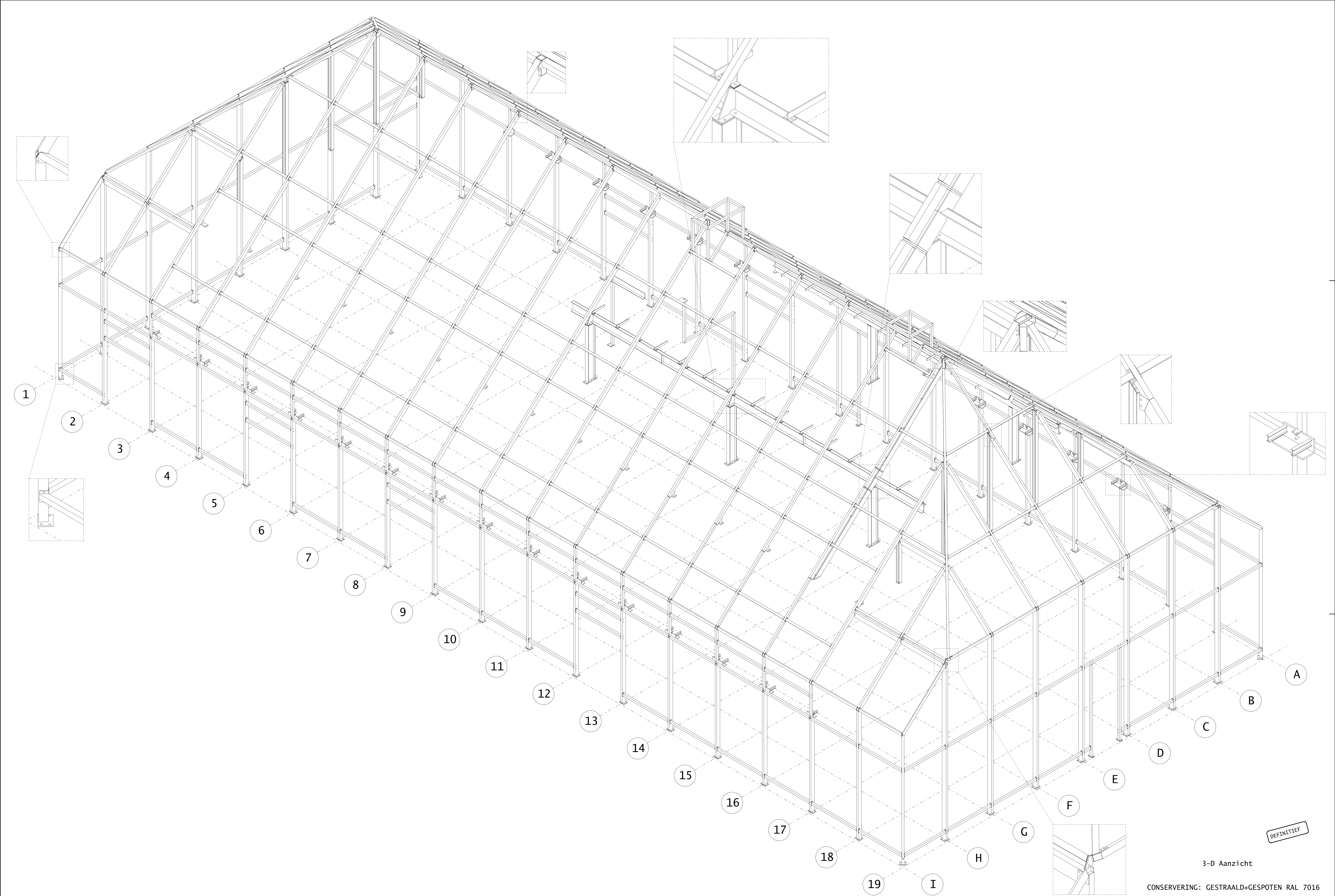
3-D Aanzicht
