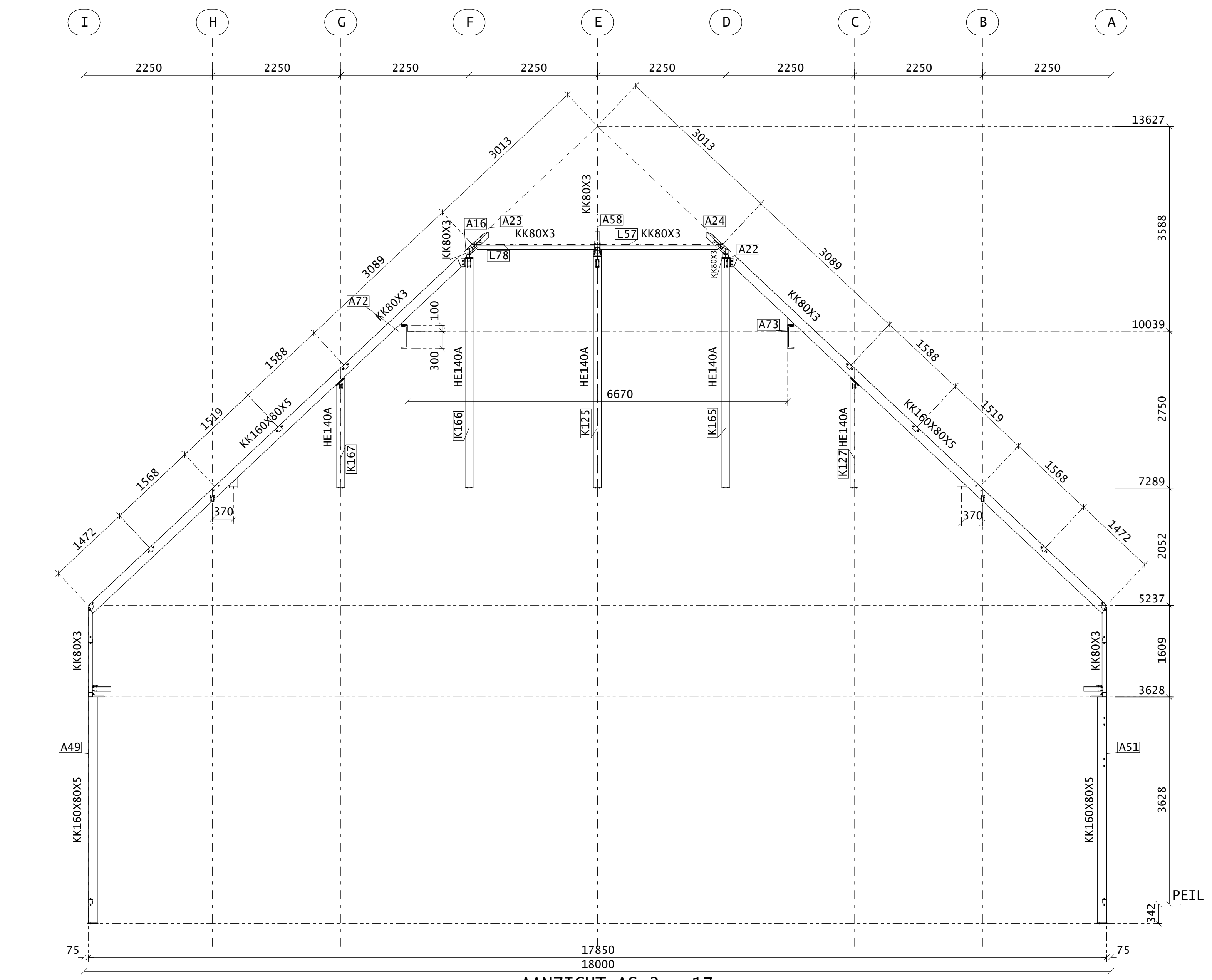
AANZICHT AS 3 + 17
