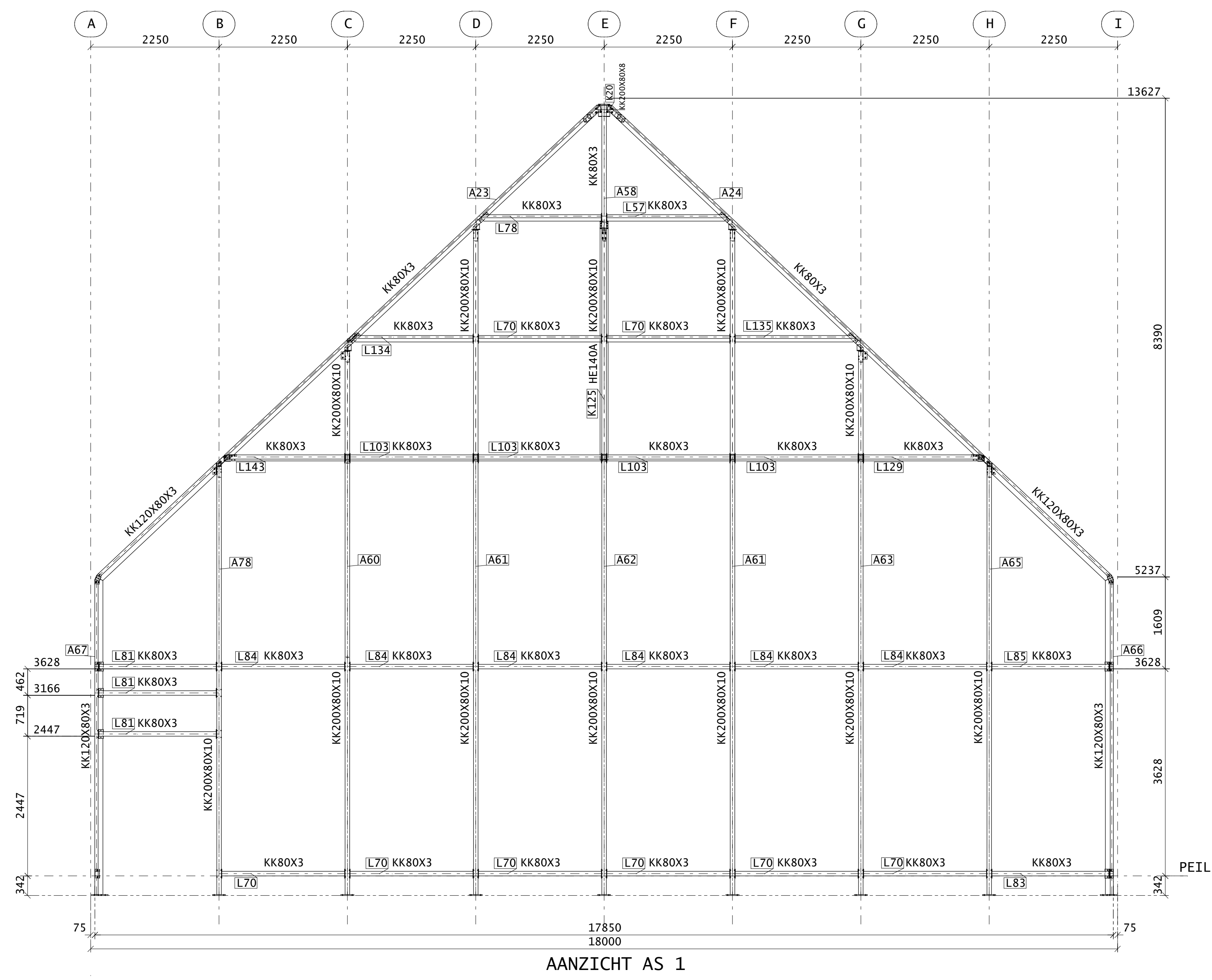
AANZICHT AS 1
