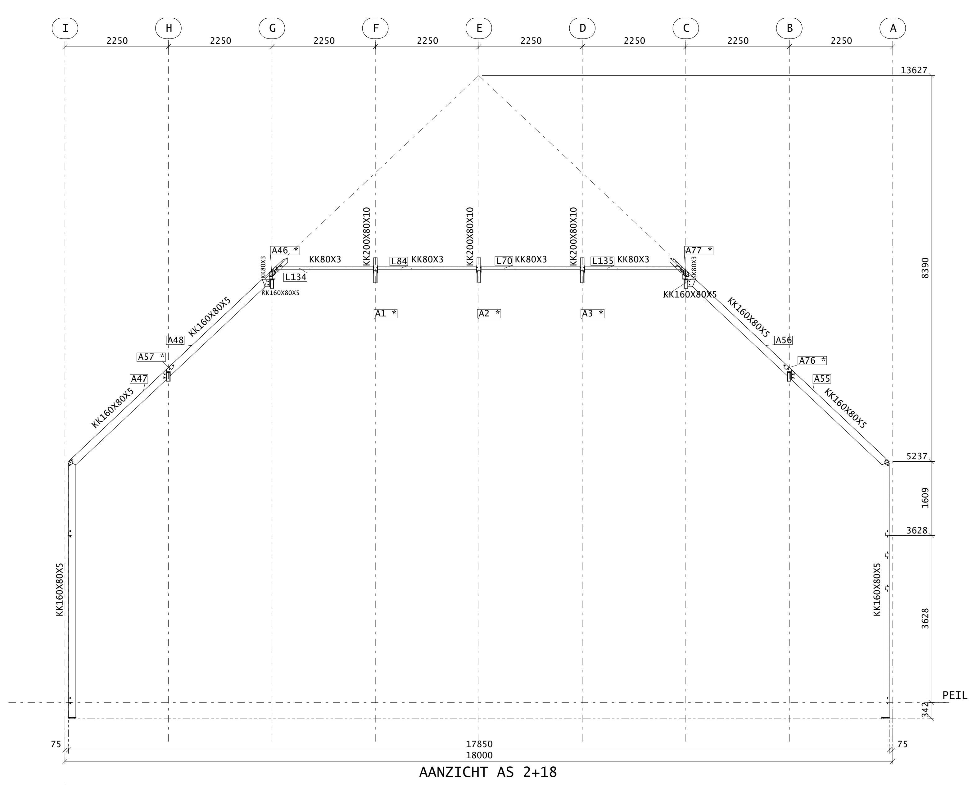
AANZICHT AS 2+18
