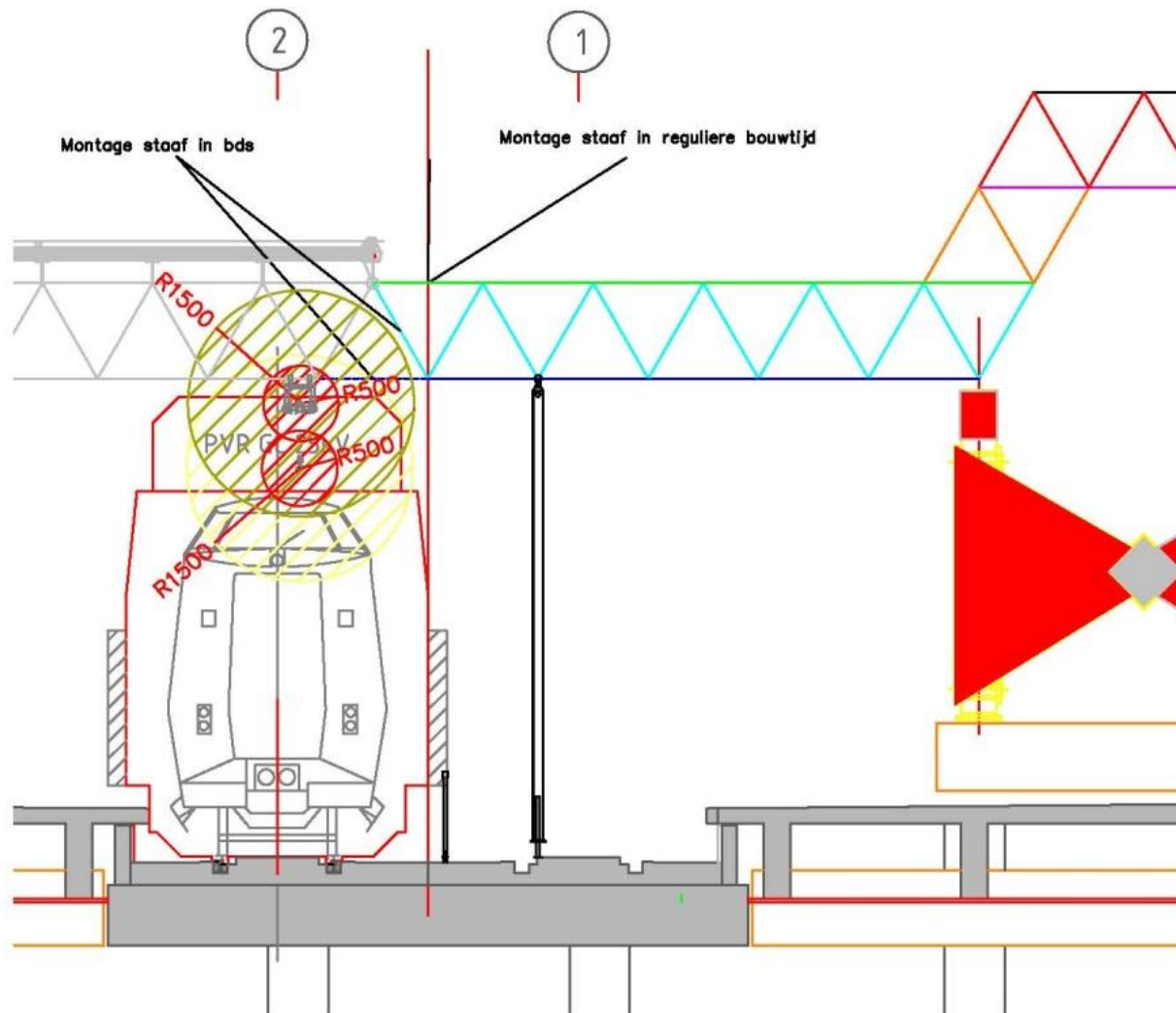
Figuur 4: Montage staven in nabijheid bovenleiding
