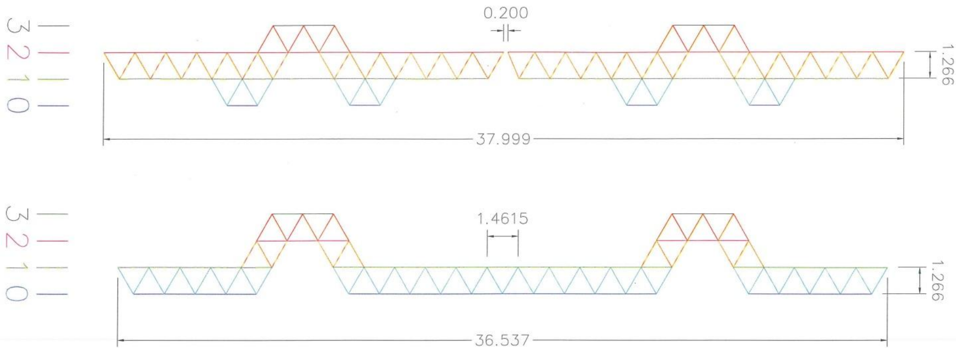
Figuur 3: Doorsnede ruimtevak werk hoog (boven) en laag (onder)
